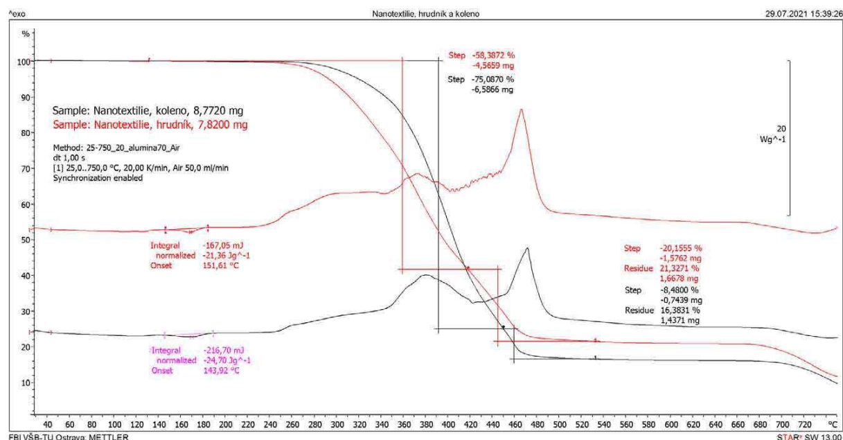
Obr. 3 TGA a DSC analýza vzorků
