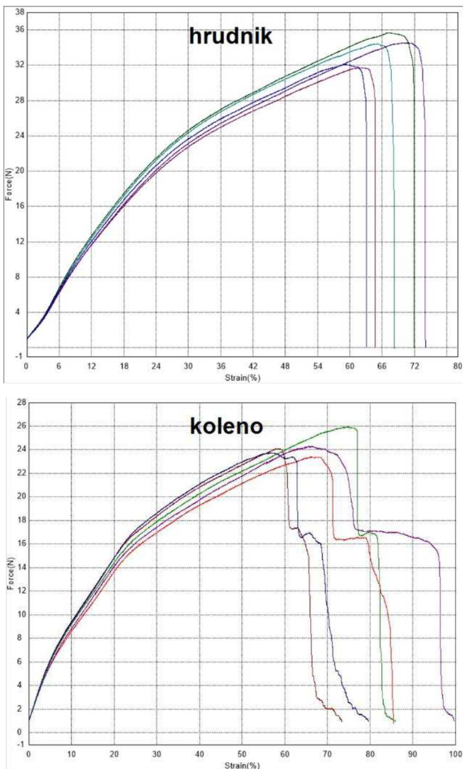
Obr. 2 Graf trhání
