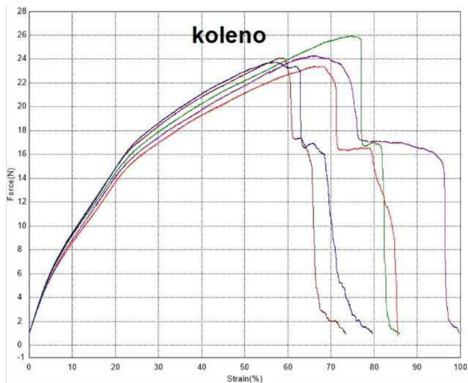
Obr. 2 Graf trhání
