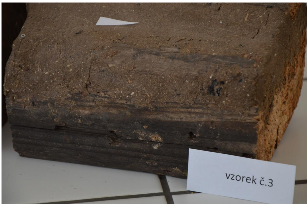
Obr. 20 Vzorek č. 3 – detail tmelení, na povrchu patrné drobné praskliny
