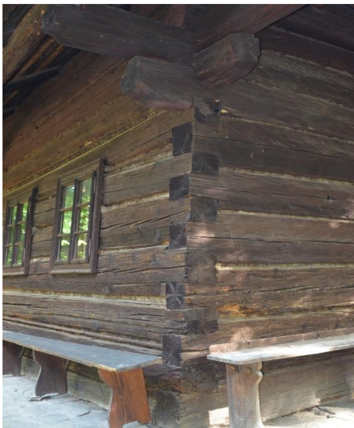
Obr. 21b Chalupa z Velkých Karlovic – Miloňova, pohled na Z stěnu s roubením poškozeným prostřednictvím výsušné trhliny
