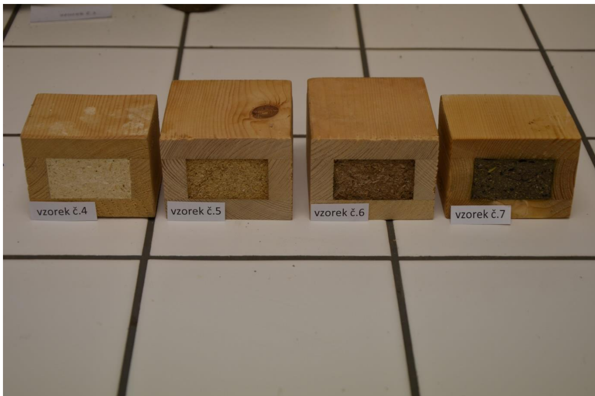
Obr. 11 Barevné vzorky kaseinových tmelů vzorek č. 4, 5, 6, 7 (vzorky barevnosti: 4 – bez patinace – smrkové piliny, 5 – dubové piliny, 6 – smrkové piliny s přidavkem barevného hnědého pigmentu, 7 – smrkové piliny s přidavkem dřevního popela)
