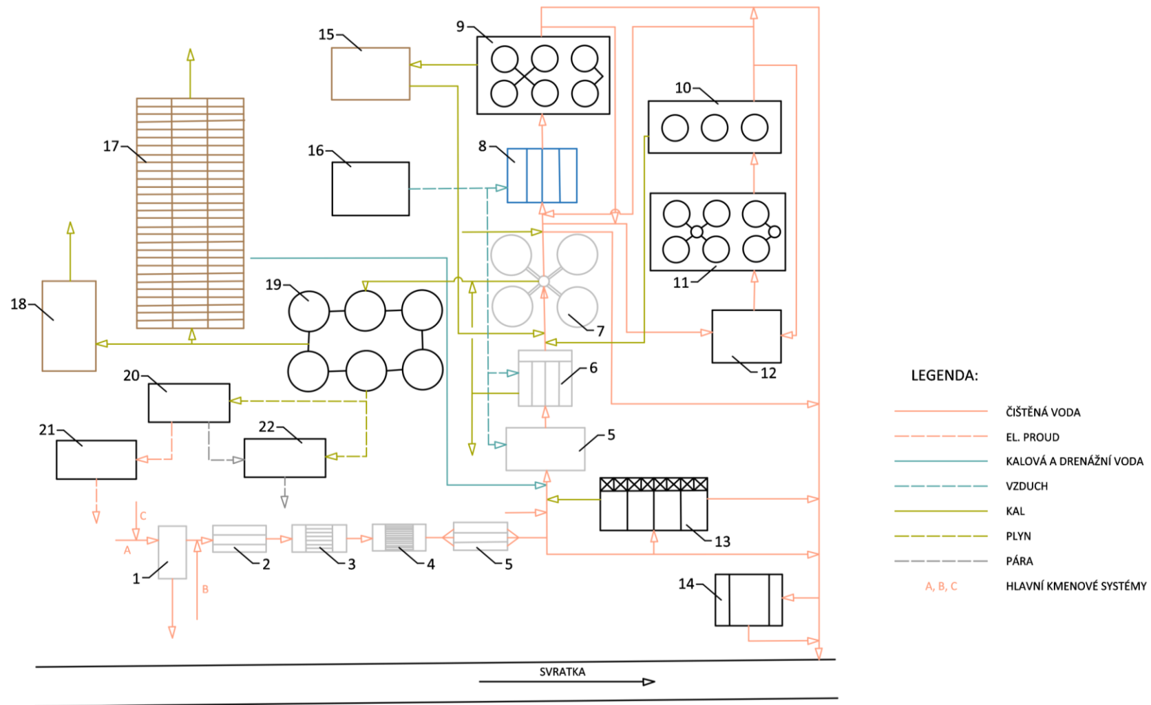
Obr. 4.262: Technologické schéma (linka) brněnské ČOV k roku 1972: 1 – přepadová komora, 2 – lapač štěrku, 3 – hrubé česle, 4 – jemné česle, 5 – lapák písku, 5 – hlavní čerpárna, 6 – lapák tuku, 7 – sedimentační nádrže, 8 – aktivační nádrže, 9 – dosazovací nádrže, 10 – dosazovací nádrže, 11 – biologické filtry, 12 – čerpárna na filtry, 13 – dešťové nádrže, 14 – povodňová čerpárna, 15 – kalová čerpárna, 16 – dmýchárna, 17 – kalová pole, 18 – humusárna, 19 – vyhnívací komory, 20 – elektrárna, 21 – rozvodna, 22 – teplárna. Schéma Radka Račoch a Michaela Mrvová, 2021 (upraveno dle: poskytnuté projektové dokumentace BVaK).
