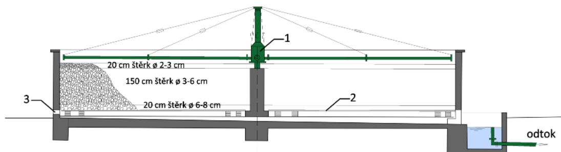
Obr. 4.248: Řez nejrozšířenějším typem biofiltru: 1 – otáčivý skrápěč, 2 – propustný rošt, 3 – větrací otvory, uvnitř konstrukce – filtrační náplň (písek, štěrk, směs různých frakcí), na obrázku znázorněn jeden příklad základní skladby filtrační náplně s průměry zrn materiálů (frakcemi). Schéma Radka Račoch a Michaela Mrvová, 2021.
