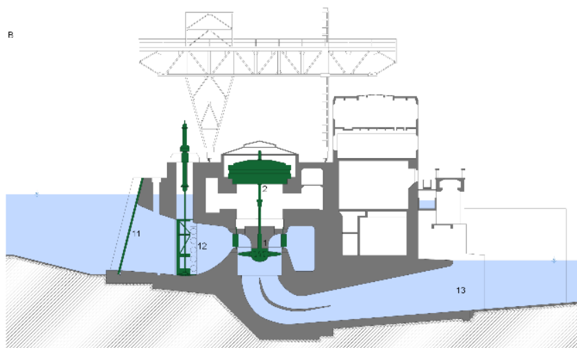
Obr. 4.140: MVE Střekov – podélný řez. Schéma Radek Mišanec, 2021 (upraveno dle: plánové dokumentace).
