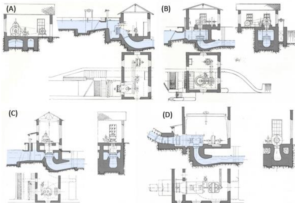
Obr. 4.177: Přívod vody na turbínu: (A) a (B) kašna; (C) betonová spirála; (D) kotlový přívod. Schéma Radka Račoch, 2021 (upraveno dle: Nechleba, 1962)
