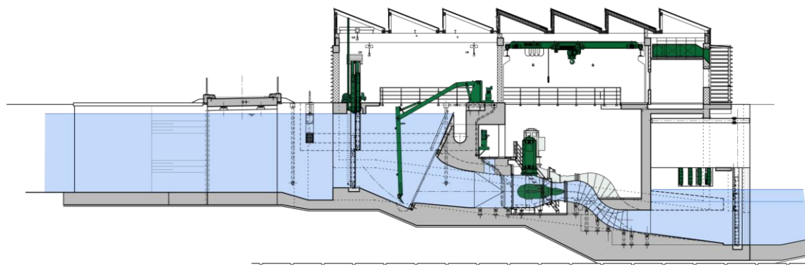
Obr. 4.136: MVE Železný Brod – podélný řez strojovnou (převzato z: Aquatis, a.s.).
