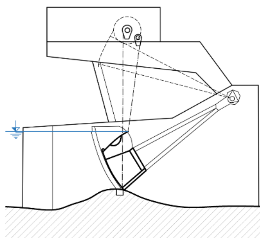
Obr. 4.109: Segmentový jez. Schéma Radka Račoch a Michaela Mrvová, 2021 (upraveno dle: Gabriel a kol., 1989). Vpravo segmentový jez v Přerově. Foto Archiv VUT, 2019.
