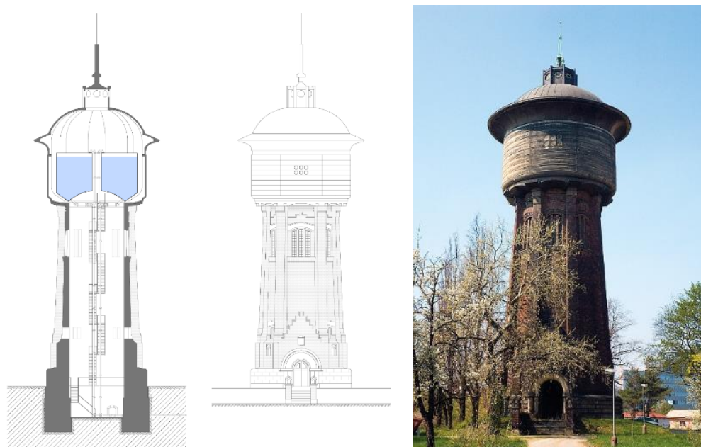
Obr. 4.220: Praha-Michle – secesní věžový vodojem Zelená Liška s válcovou ocelovou nádrží o objemu 1 200 m 3 byl součástí vršovické vodárny. Byl postaven v letech 1906–1907 podle návrhu Karla Kresse
