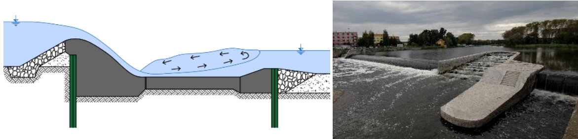
Obr. 4.102: Vlevo pevný betonový jez. Schéma Radka Račoch a Radek Bachan, 2021 (upraveno dle: Gabriel a kol., 1989). Vpravo jez v Břeclavi. Foto archiv VUT, 2019.
