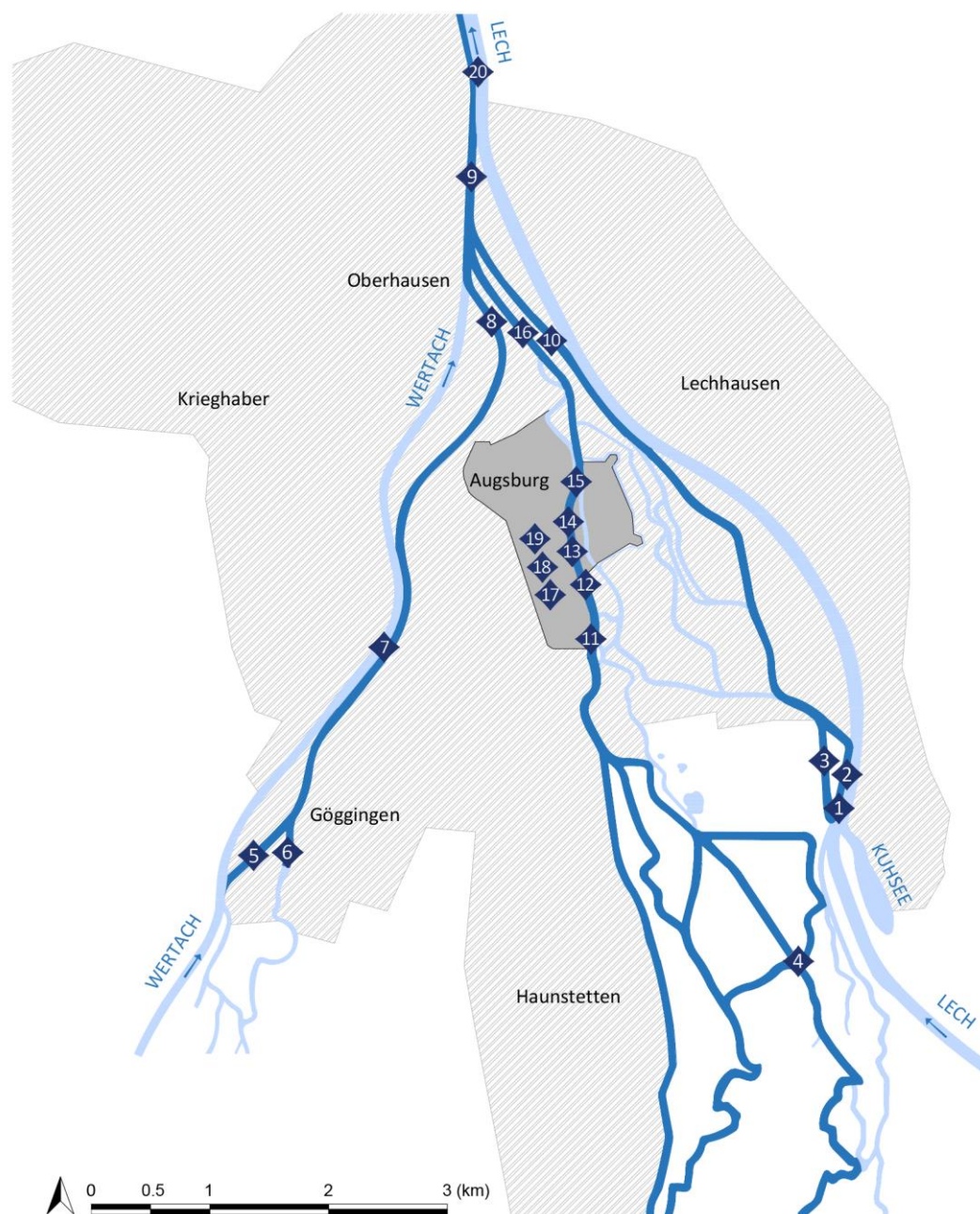
Obr. 3.1: Augsburg, schéma vodohospodářského systému. Součásti systému: 1 – jez Hochablass je vzdouvacím dílem pro většinu městských kanálů, současná podoba pochází z let 1911–1912 s výjimkou několika obnovených částí; 2 – kanály řeky Lech jsou poprvé zmiňovány v roce 1276, dodávaly vodu řemeslným podnikům, poháněly vodní kola, později vodní turbíny; 3 – Galgenblass (propust) – nejdůležitější křížení vodních toků, díky kterému jsou voda pitná a užitková vedena odděleně; 4 – vodárna u Červené brány – soubor tří vodárenských věží s čerpací stanicí zásoboval město od roku 1416 a je považován nejstarší známý vodárenský systém ve střední Evropě, jeho čerpací stroje pracovaly do roku 1880; 5 – dolní kašna provozovaná asi od roku 1500; 6 – kašna u Ptačí brány (Vogeltor) z roku 1538, roku 1774 byla hradební věž přeměněna na vodárenskou; 7–9 – soubor tří monumentálních kašen završených bronzovými sochami a sousošími: Augustova kašna z roku 1594, Merkurova z roku 1599 a Herkulova z roku 1602; 10 – městská jatka z roku 1609 s inovativním využitím vody z kanálu, jež stavbou prochází, k chlazení masa a likvidaci odpadu; 11 – vodárna u jezu Hochablass, počátek moderního zásobování města vodou, z let 1879–1880;
