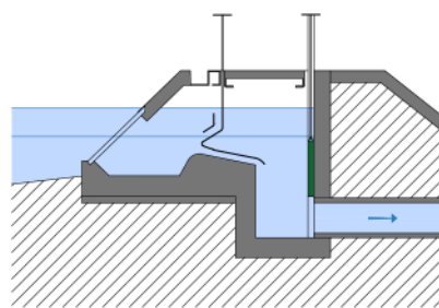
Obr. 4.209: Břehové jímadlo: 1 – vodní tok, 2 – česle, 3 – norná stěna, 4 – měrný práh, 5 – šachta, 6 – stavidlo, 7 – hráz, 8 – odběr vody potrubím. Schéma Radek Míšanec, 2021 (upraveno podle: Milerski 2005).
