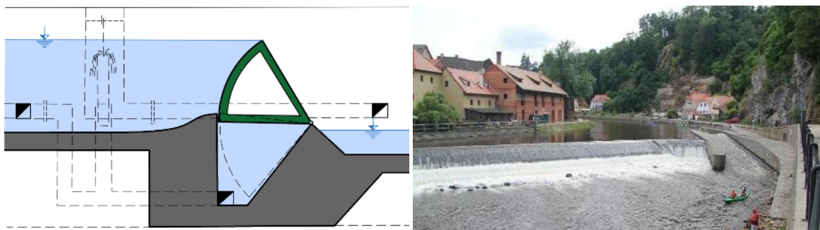
Obr. 4.111: Sektorový jez. Schéma Radka Račoch a Michaela Mrvová, 2021 (upraveno dle: Jermář, 1956). Vpravo sektorový jez na Vltavě v Českém Krumlově. Foto Archiv VUT, 2019.
