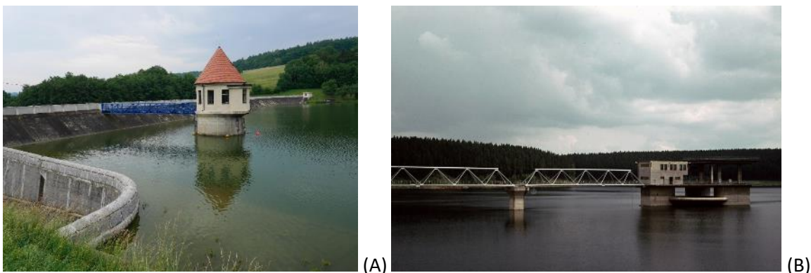
Obr. 4.208: Samostatně stojící sdružené objekty pro odběry vody z nádrží: (A) Přehrada Fryšták, samostatně stojící sdružený objekt výpustí a vodárenských odběrů se strojovnou pro ovládnání uzávěrů výpustí v horní části. Odběr vody zajišťují dvě potrubí ve dvou úrovních. Součástí vodního díla je také úpravná, situovaná pod hrází přehrady. Foto Michaela Ryšková, 2020; (B) Vodní dílo Švihov, zdroj surové vody pro úpravnu vody Želivka. Samostatně stojící sdružený odběrný objekt hráze. Odběr vody je zajištěn dvěma odběrnými pilíři s možností pěti etážových odběrů, sahající až na dno nádrže, zakončenou v koruně nouzovým přepadem. Voda je vedena do čerpací stanice u paty nádrže a dále do úpravny vody (Parkán a Pěkný, 2012).
