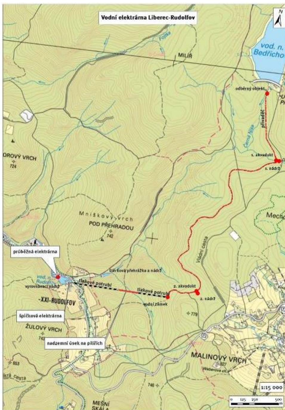
Obr. 5.6: Rudolfov – schéma vodního díla (převzato z: Freiwillich, 2019).
