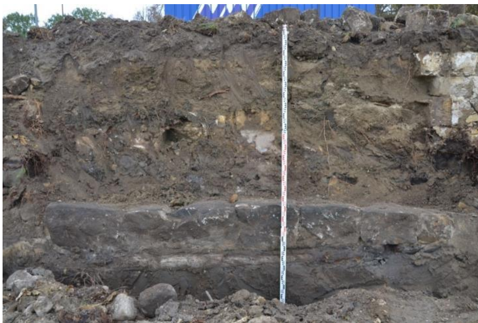
Obr. 4.54: Holany, Holanský rybník – konstrukce hráze s opevněním návodního líce, pískovcové zdivo je založeno na trémovém roštu z počátku 16. století. Foto Miroslav Kolka, 2018.
