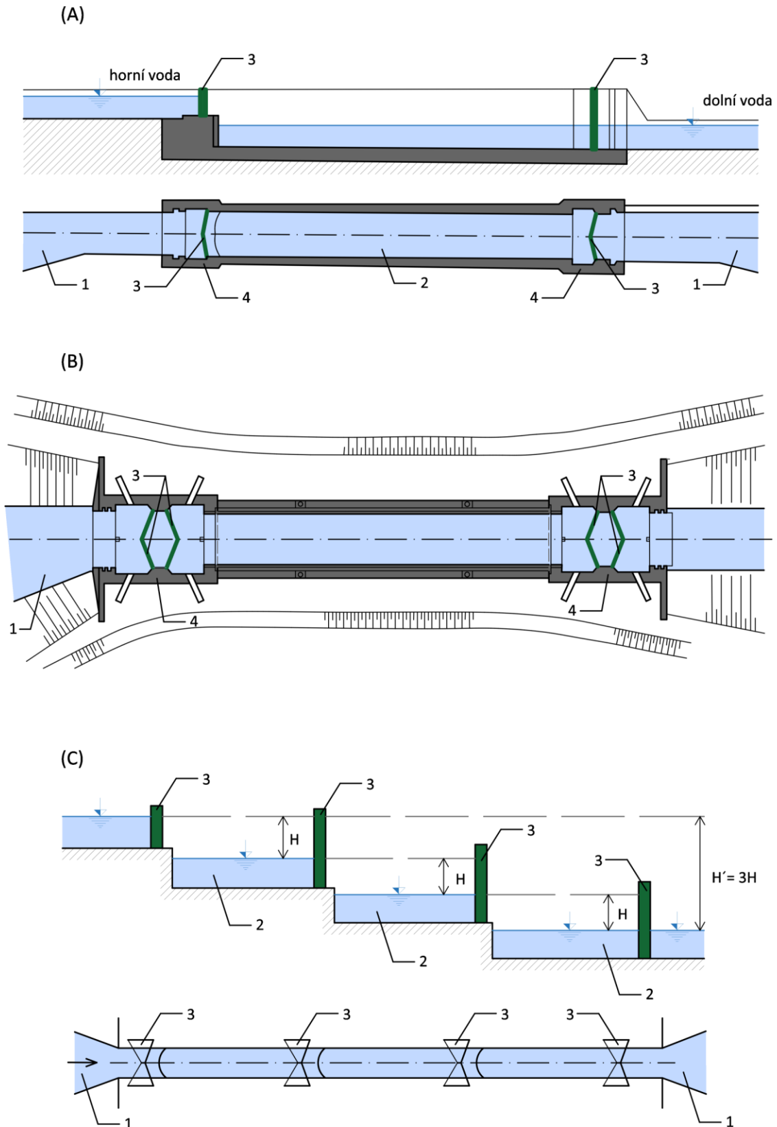
Obr. 4.77: (A) Schéma jednoduché plavební komory; (B) Komora se zdvojenými vraty; (C) Schéma plavební komory víceúrovňové; 1 – rejda, 2 – vlastní komora, 3 – vrata komory, 4 – zhlaví. Schéma Radka Račoch, Radek Bachan a Michaela Mrvová, 2021 (upraveno dle: VŠB – TUO, 2013).
