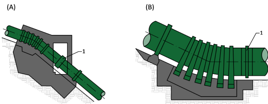
Obr. 4.155: Příklady konstrukce kotevních bloků: (A) uzavřený typ; (B) otevřený typ; 1 – dilatační kus. Schéma Radka Račoch a Radek Bachan, 2021 (upraveno dle: Broža a kol., 1990).
