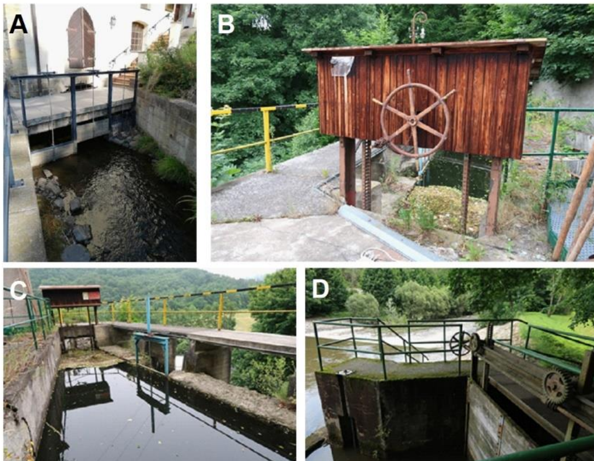
Obr. 4.94: Detaily ovládacích objektů: (A) Chrudim dřevěná, ručně ovládaná stavidla; (B) Weissshuhnův kanál, stavidlo ovládané původně ručně přebudované na elektropohon; (C) tamtéž pravobřežní jalový odtok ovládaný hydraulicky; (D) mechanismus pro ruční ovládání stavidel z boku. Foto Radka Račoch, 2021.
