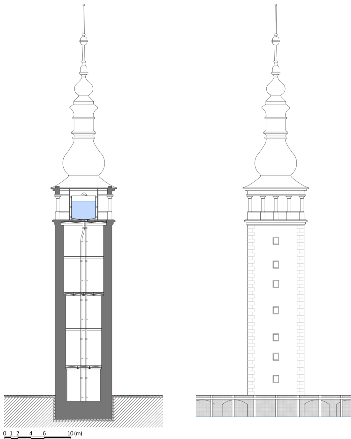
Obr. 4.189: Praha – Staroměstská vodárenská věž, vybudovaná pro potřeby staroměstské vodárny. Schéma Radek Míšanec, 2021 (upraveno dle: plán z APVK, nesignováno).
