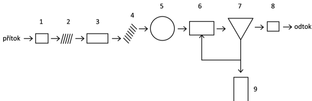
Obr. 4.234: Blokové schéma technologické linky čistírny odpadních vod: 1 – lapák štěrku, 2 – česle, 3 – lapák písku a tuků, 4 – zdvih, 5 – usazovací nádrž, 6 – biologický reaktor, 7 – dosazovací nádrž, 8 – terciární dočištění, 9 – kalové hospodářství. Schéma Radka Račoch a Radek Bachan, 2021 (upraveno dle: archiv VÚV).
