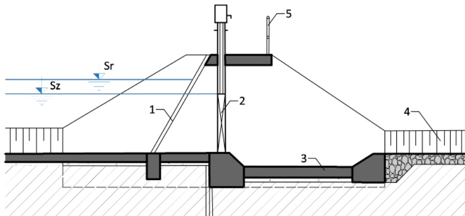
Obr. 4.57: Schéma stavidla: 1 – česle, 2 – stavidlo, 3 – vývar, 4 – odpad, 5 – manipulační lávka, Sz – hladina zásobního prostoru, Sr – hladina ovladatelného retenčního prostoru. Schéma Radka Račoch a Michaela Mrvová, 2021 (upraveno dle: Tlapák, Herynek, 2002).
