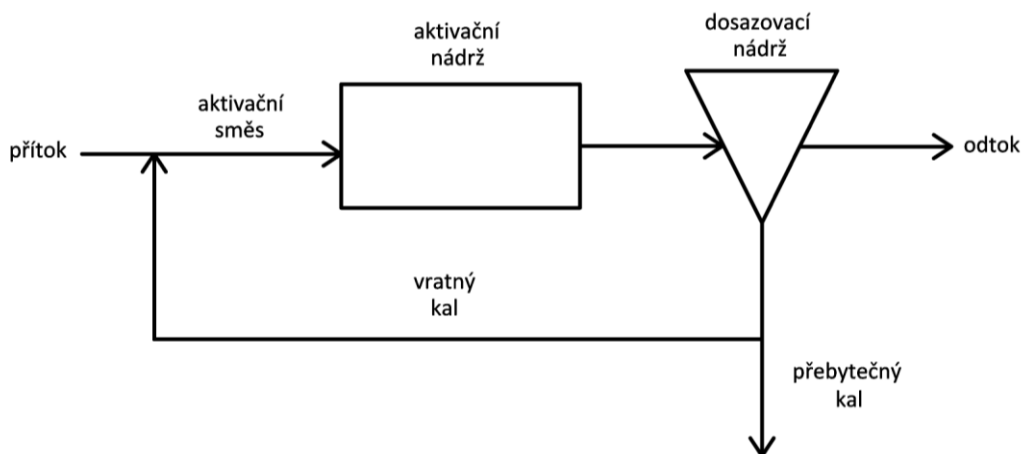
Obr. 4.249: Blokové schéma klasické aktivace. Schéma Radka Račoch a Radek Bachan, 2021 (upraveno dle: archiv VÚV).
