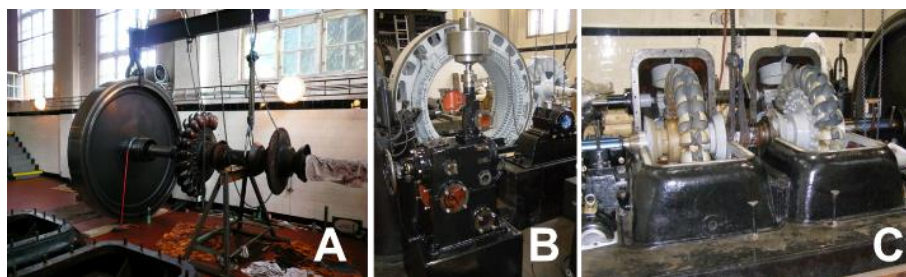
Obr. 5.9: Generální oprava turbosoustrojí MVE Rudolfov I – setrvačnick a oběžná kola dvojčité Peltonovy turbíny s částečně odmontovanými lopatkami (vlevo), generátor po renovaci a původní regulátor turbíny (uprostřed), oběžná kola a hřídel po renovaci. Foto Petr Nedomlel, 2008 (A), 2012 (B) a (C).
