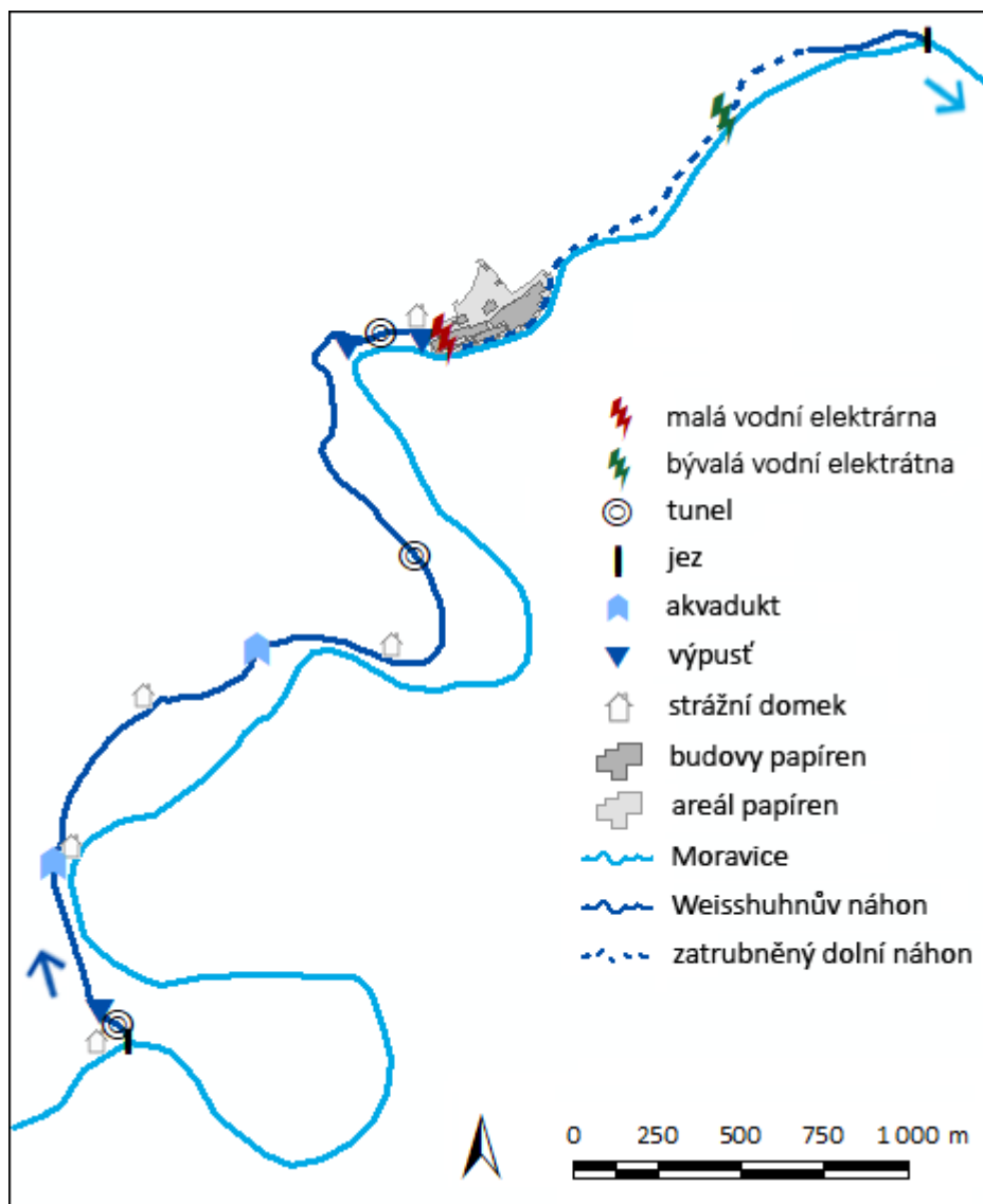
Obr. 4.182: Žimrovice – funkční celek papírny s vyznačením jednotlivých významných objektů. Schéma Radek Bachan, 2021 (upraveno dle: SOKA Opava, karton 1052, 1911 – 1914).
