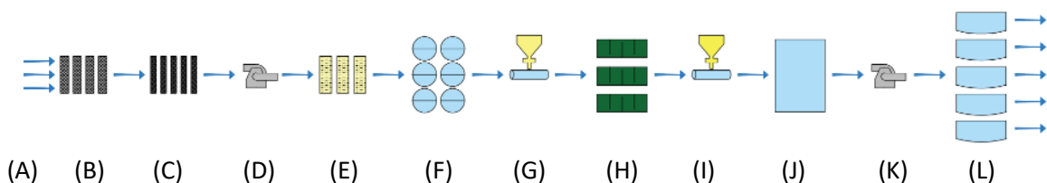
Obr. 4.197: Schéma úpravy vody v úpravně vody Podolí: (A) odběr surové vody v Vltavy; (B) hrubé česle v jímacím objektu na Veslařském ostrově; (C) jemné česle v objektu úpravní; (D) čerpání surové vody do
