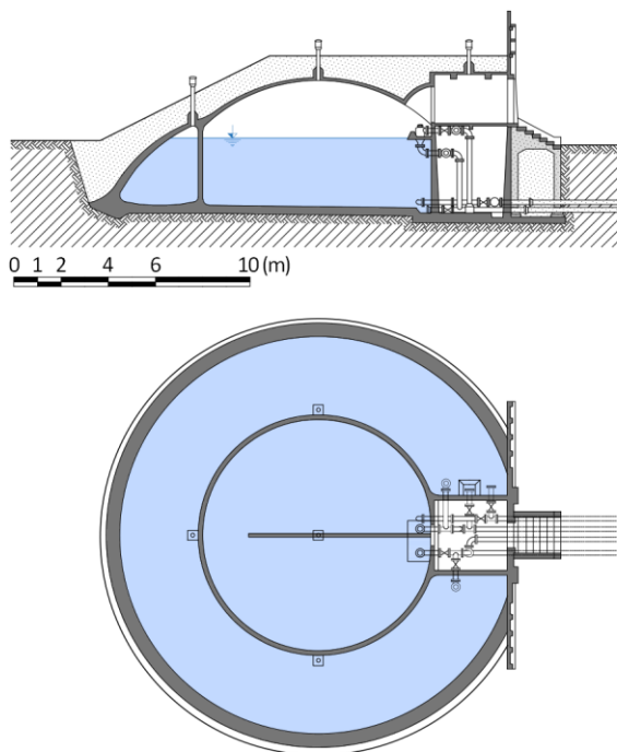
Obr. 4.214: Zemní vodojem železobetonový sférického tvaru. Schéma Radek Míšanec, 2021 (upraveno dle: Klír a Klokner, 1923).
