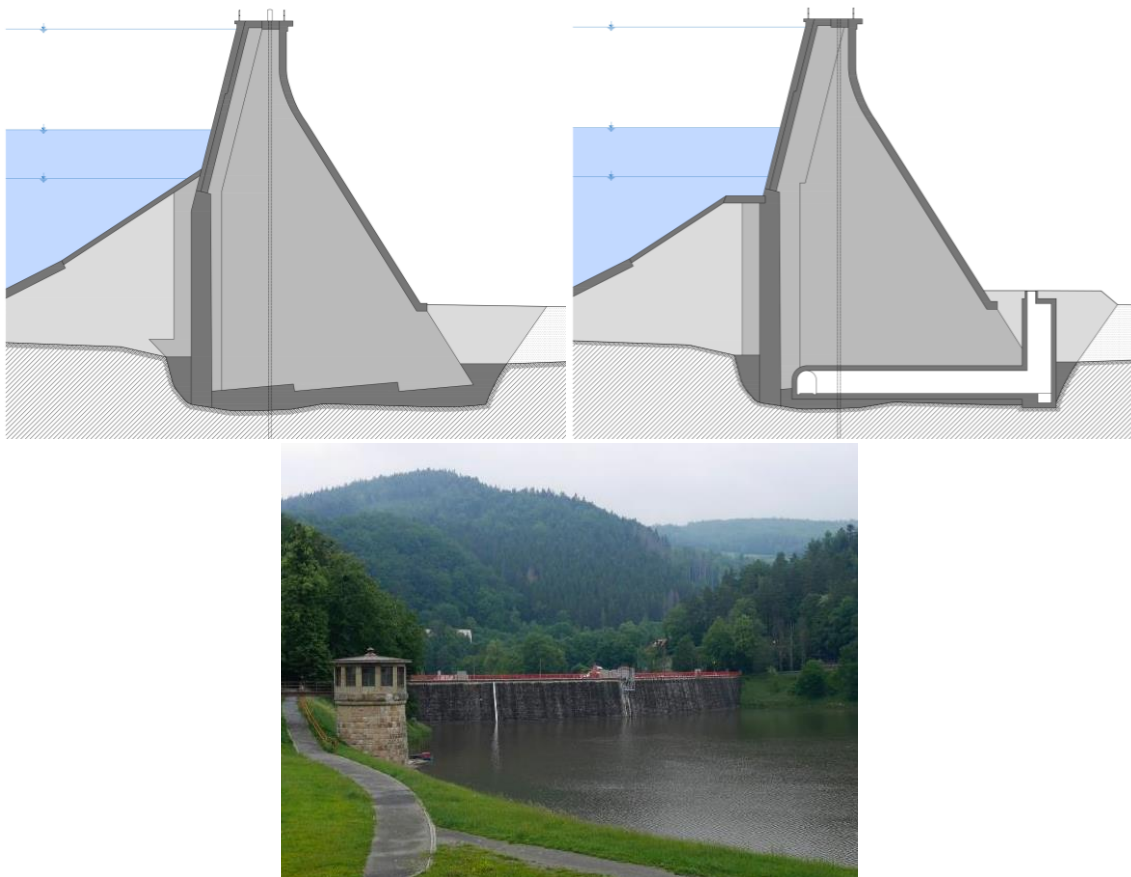
Obr. 3.8: Přehrada Bystřička (1908–1912), řez hrázi před a po rekonstrukci. Schéma Radek Míšanec, 2021 (upraveno dle: PMO, 2019a). V letech 2004–2005 byla provedena celková rekonstrukce hráze pro zvýšení protipovodňového účinku a navýšení bezpečnosti při extrémních povodních. Mimo jiné byla vybudována injekční štola v tělese hráze, zesílena injekční clona, proveden nový drenážní a odvodňovací systém a
