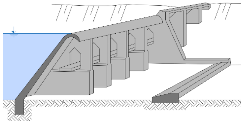
Obr. 4.103: Členěný pilířový jez. Schéma Radek Míšanec, 2021 (upraveno dle: Gabriel a kol., 1989).
