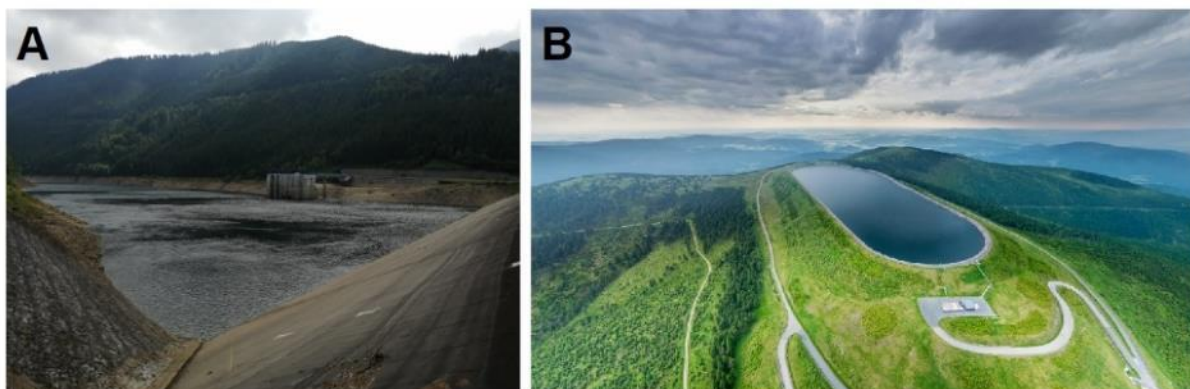
Obr. 3.21: PVE Dlouhé Stráně: (A) dolní nádrž; (B) horní nádrž; příklad údolní a vrcholové nádrže s kontroverzní krajinnou/urbanistickou hodnotou a velkým vlivem na vzhled dané lokality. U horní nádrže došlo k významnému vlivu na panorama Hrubého Jeseníku díky odtěžení vrcholu hory a jejího zarovnání („odseknutí“). Foto (A) David Honek, 2019, (B) převzato z: Dlouhestrane.cz, 2021).
