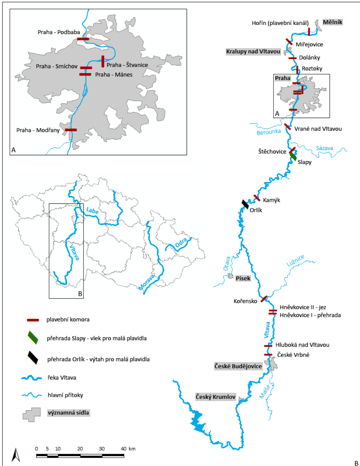
Obr. 4.114: Vltavská vodní cesta. Schéma Radek Bachan, 2021.
