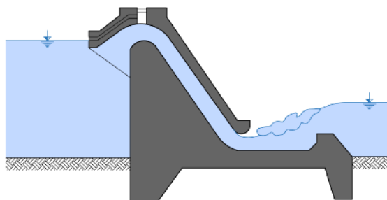
Obr. 4.104: Násoskový jez. Schéma Radka Račoch a Radek Bachan, 2021 (upraveno dle: Průcha, 1980).
