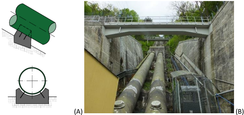
Obr. 4.154: Konstrukce podpěrného bloku: (A) schéma Radka Račoch a Radek Bachan, 2021 (upraveno dle: Broža a kol., 1990); (B) PVE Štěchovice – tlakové potrubí s podpěrnými a kotevními bloky. Foto VUT v Brně, FAST, 2019.
