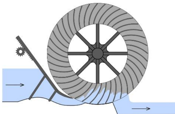
Obr. 4.170: Vodní kolo Ponceletovo. Schéma Radka Račoch a Michaela Mrvová, 2021 (upraveno dle: Hýbl 1922; Štěpán a kol., 2008; NM, 2021).
