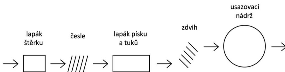
Obr. 4.235: Blokové schéma mechanické části čistírny odpadních vod. Schéma Radka Račoch a Radek Bachan, 2021 (upraveno dle: archiv VÚV).
