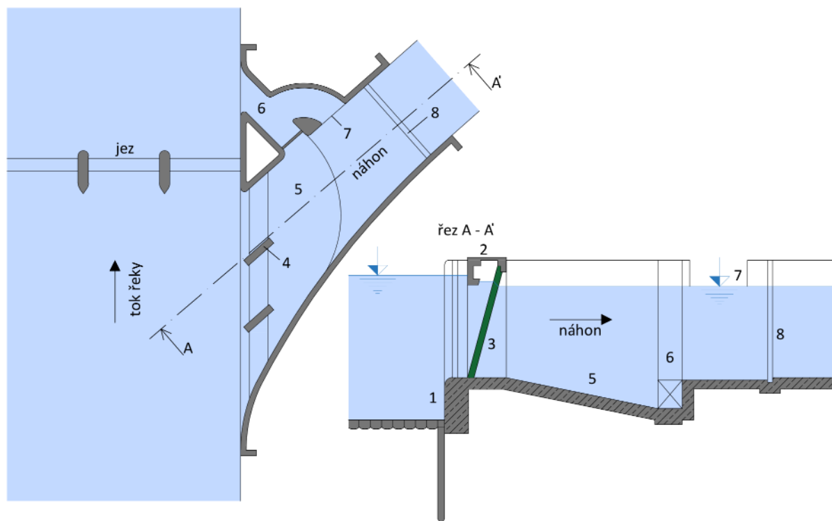
Obr. 4.142: Schéma vtokového objektu derivační VE: 1 – vtokový práh, 2 – normá clona, 3 – hrubé česle, 4 – dělící pilíř, 5 – usazovák, 6 – proplachovací kanál, 7 – boční (jalový) přepad, 8 – regulační uzávěr. Schéma Radek Míšanec, 2021 (upraveno dle: Kratochvíl, 1956).
