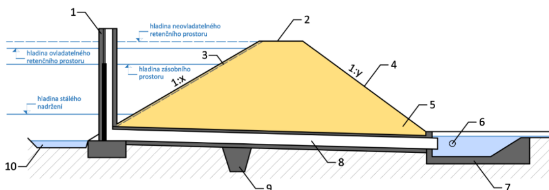
Obr. 4.43: Obecné schéma nádrže: (1) – výpustní zařízení (požerák), (2) – koruna hráže, (3) – návodní strana, (4) – vzdušná strana, (5) – patní drén, (6) – potrubní jáma, (7) – vývar, (8) – výpustné potrubí, (9) – zavazovací ostruha, (10) – mrtvý prostor. Schéma Radka Račoch a Radek Bachan, 2021 (upraveno dle: MZE, 2015).
