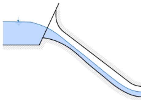
Obr. 4.33: Tunelový bezpečnostní přeliv. Schéma Radka Račoch a Radek Bachan, 2021 (upraveno dle: Broža a kol., 1987).
