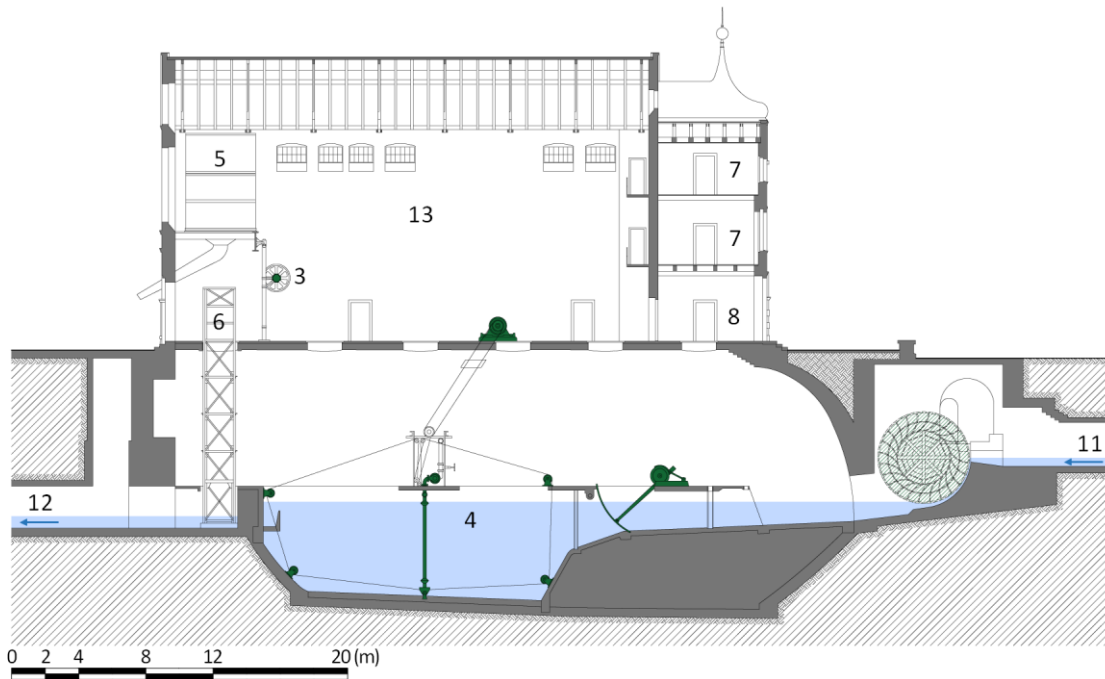
Obr. 4.260: Praha-Bubeneč – stará čistírna odpadních vod, řez hlavní budovou: 1 – strojovna, dvojice parních jednoválcových dvojčinných ležatých strojů, 2 – strojovna, odstředivá vodní čerpadla - povodňové pumpy, 3 – transmise pohonu vodních pump, 4 – lapák písku, 5 – rezervoár na písek a čistou vodu, 6 – manipulační výtah, 7 – kanceláře, 8 – chodby, schodiště atd., 9 – sociální a hygienické místnosti, 10 – laboratoře, 11 – přítok ze stok do lapáku písku, 12 – odtok z lapáku písku do sedimentačních nádrží, 13 – hala lapáku písku, 14 – kotelna a uhelna, 15 – dva sdružené plamencové kotle typu Cornisch, 16 – skladovací prostory, archivy atd., 17 – rozvodna a skladovací prostor, 18 – pístová vodní čerpadla, 19 – rezervoár na kaly, 20 – komín k odvodu spalin od kotlů, 21 – ventilační komín, odvod pachů ze stok. Schéma Radek Míšanec, 2021 (upraveno dle: archivní projektové dokumentace).
