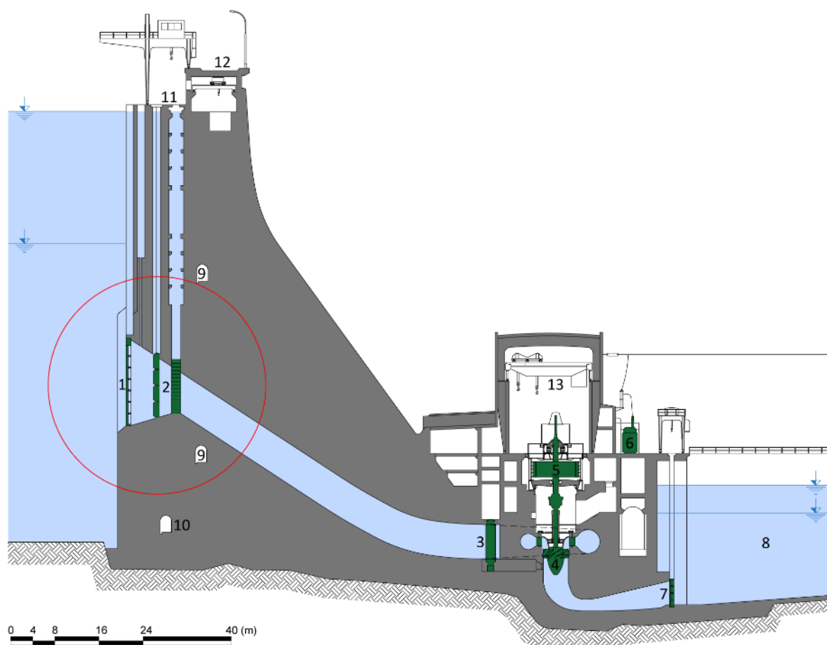
Obr. 4.145: VD Orlík – podélný řez elektrárenským blokem: 1 – česle, 2 – revizní a provozní uzávěr, 3 – provozní uzávěr před turbínou, 4 – Kaplanova turbína, 5 – generátor, 6 - blokový transformátor, 7 –
