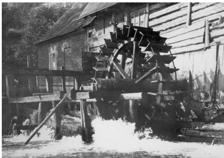
Obr. 4.167: Hřebenáč jednookružní. Foto Jan Popelka, podsběrka fotografie-pozitivů, Regionální muzeum ve Vysokém Mýtě, inv. č. 22D-4842.
