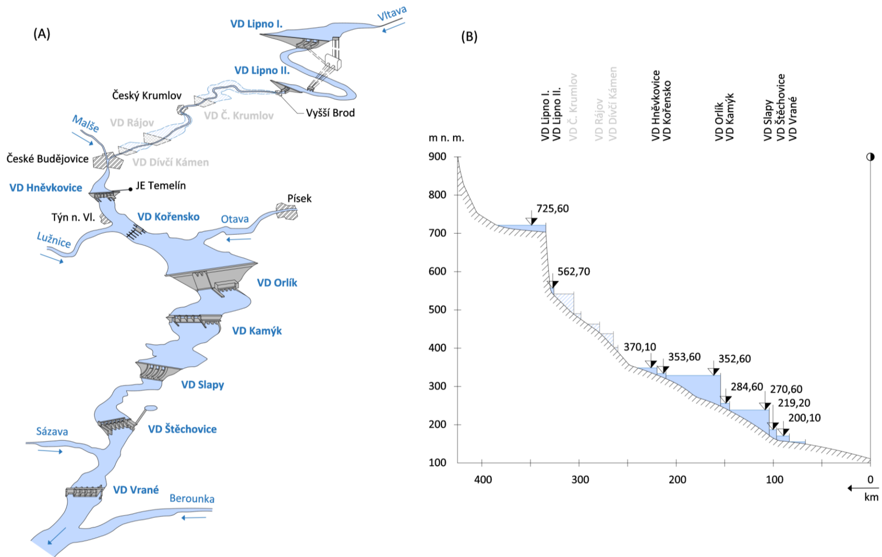
Obr. 4.37: (A) Vltavská kaskáda; (B) Podélný profil. Schéma Radek Míšanec a Radka Račoch, 2021 (upraveno dle: Dvořák a kol., 1969, Broža a kol., 2005).
