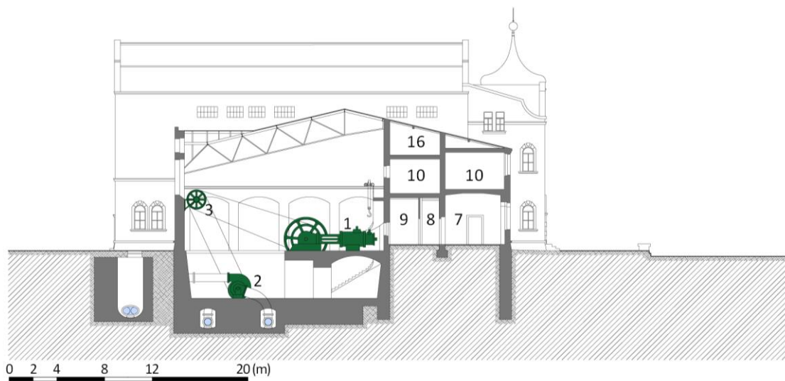
Obr. 4.261: Praha-Bubeneč – stará čistírna odpadních vod, řez hlavní budovou: 1 – strojovna, dvojice parních jednoválcových dvojčinných ležatých strojů, 2 – strojovna, odstředivá vodní čerpadla - povodňové pumpy, 3 – transmise pohonu vodních pump, 4 – lapák písku, 5 – rezervoár na písek a čistou vodu, 6 – manipulační výtah, 7 – kanceláře, 8 – chodby, schodiště atd.; 9 – sociální a hygienické místnosti, 10 – laboratoře, 11 – přítok ze stok do lapáku písku, 12 – odtok z lapáku písku do sedimentačních nádrží, 13 – hala lapáku
