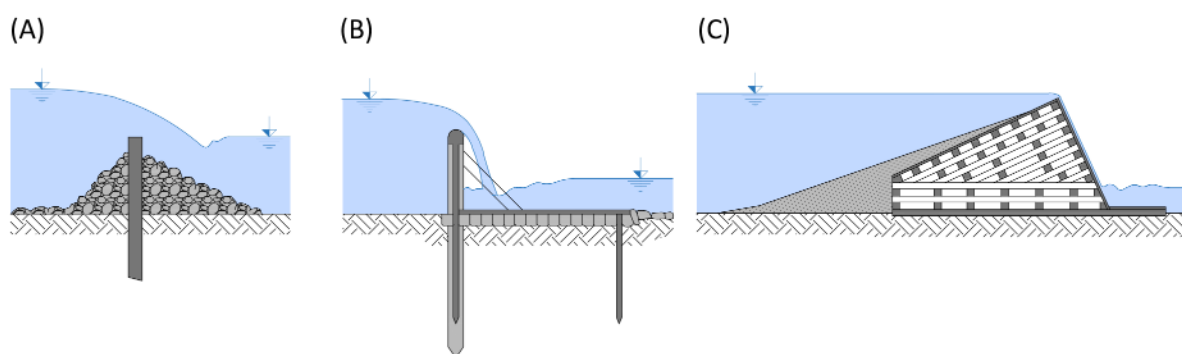
Obr. 4.98: Ukázka typů dřevěných jezů: (A) Hradicí konstrukce s dřevěnou pilotovou stěnou doplněnou stabilizačním kamenným materiálem; (B) Hradicí konstrukce stabilizovaná dřevěnými vzpěrami; (C) Jezová konstrukce srubového typu. Schéma Radek Míšanec, 2021 (upraveno dle: Průcha, 1980).
