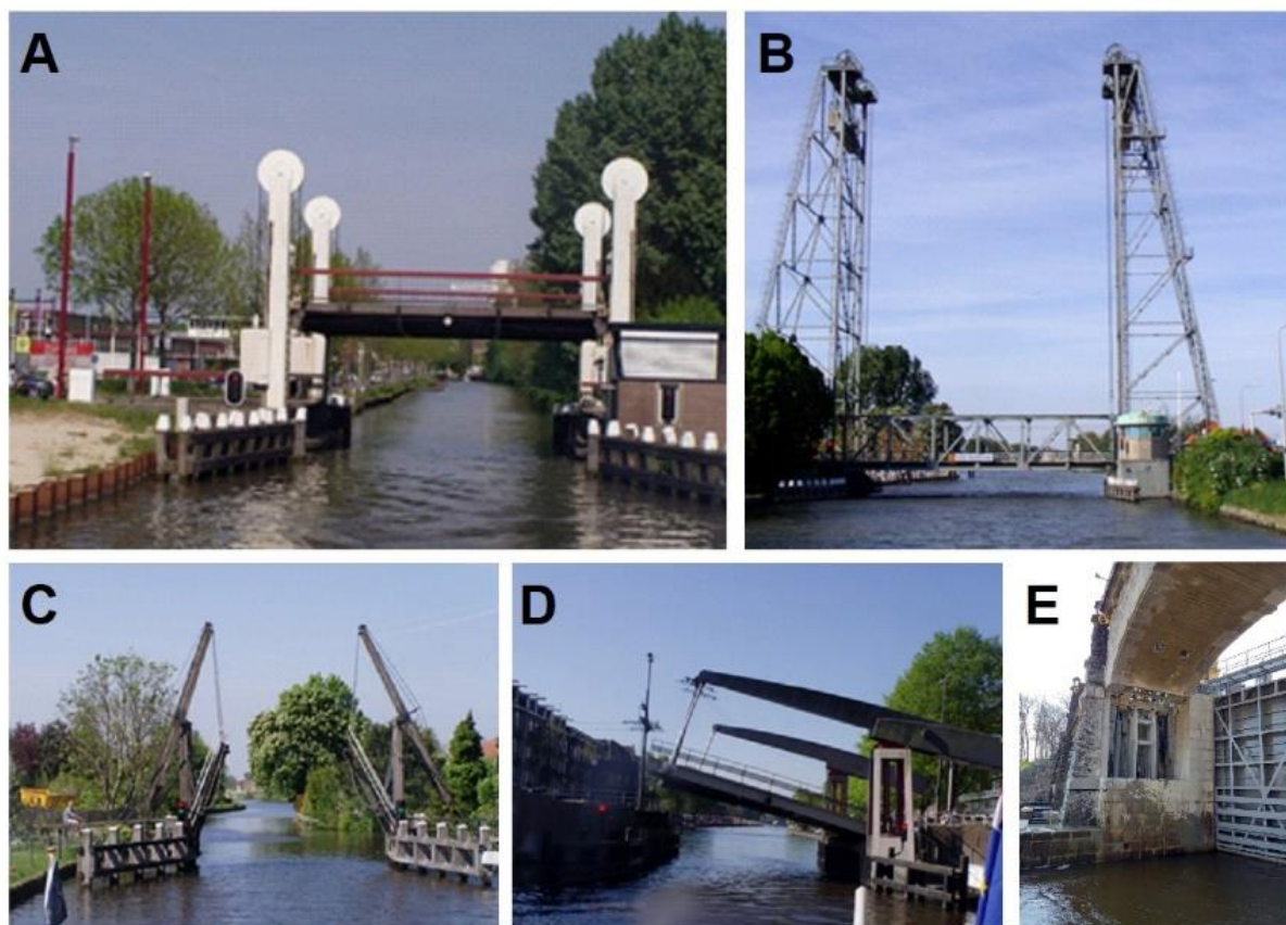
Obr. 4.83: Zvedací mosty různých konstrukcí: (A) a (B) s protizávažím, zvedané s vozovkou v horizontální poloze; (C), (D) vahadlové; (E) hydraulicky ovládaný most na rekonstruovaném zdymadle Hořín. Foto (A) – (D) Vít Forejtník, 2007 (Holandsko); (E) Otakar Hrdlička, 2021.
