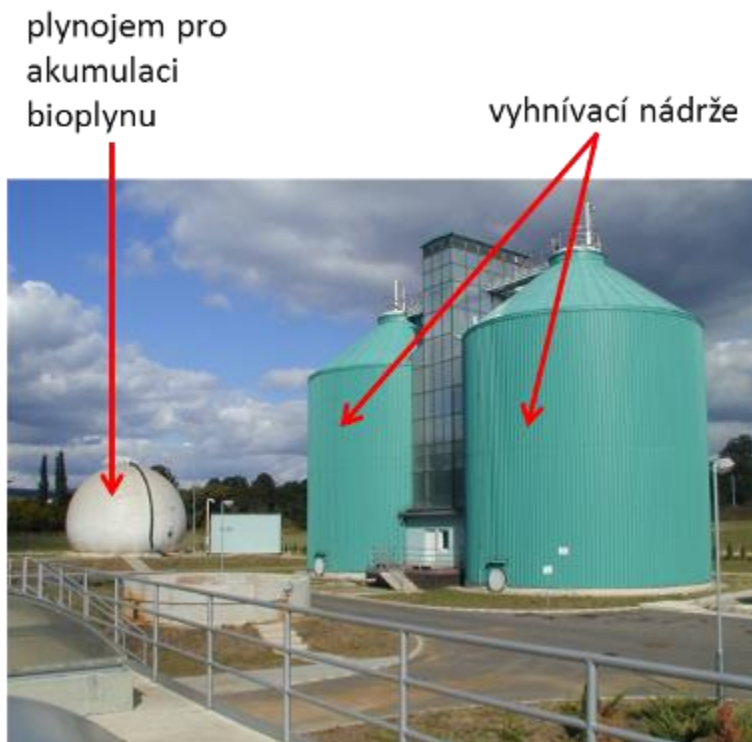
Obr. 4.256: Kalové hospodářství na ČOV – vyhnívací nádrže s bioplynem (převzato z: archiv VÚV).
