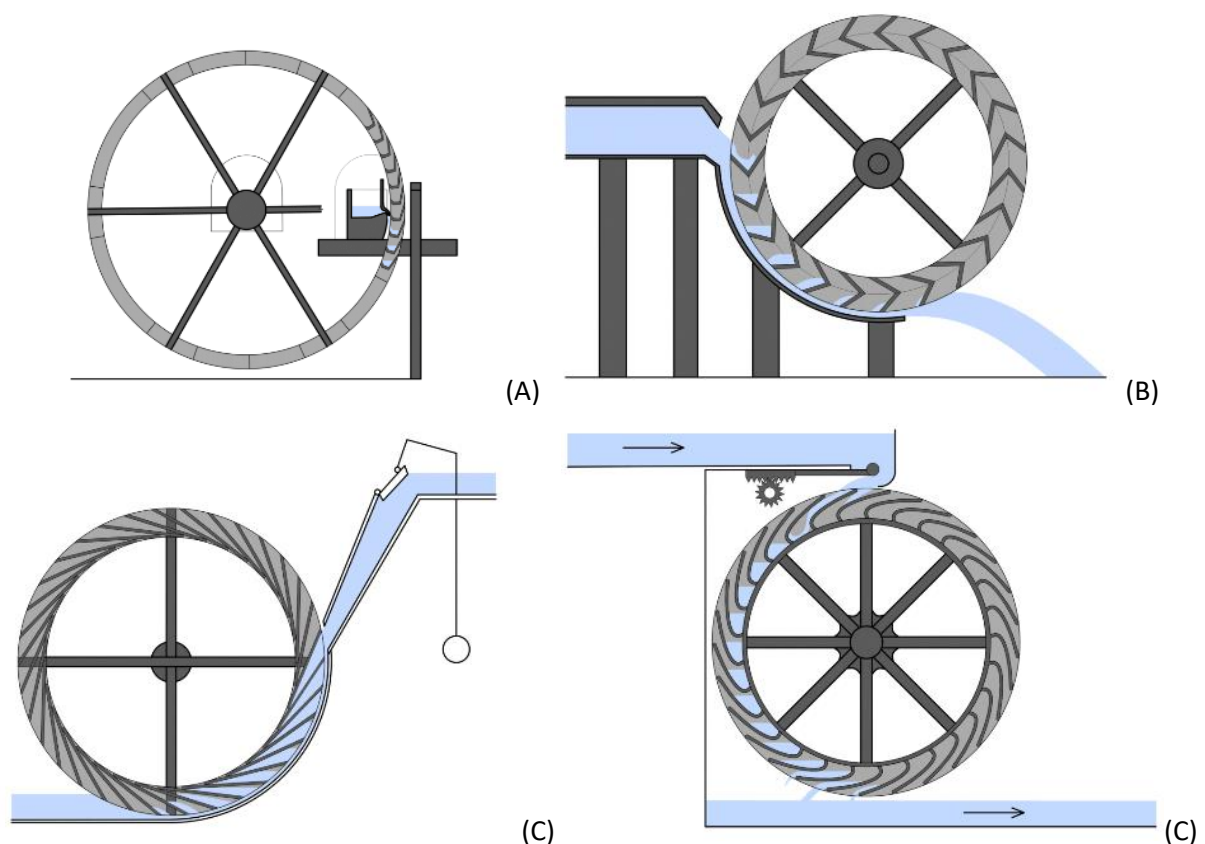
Obr. 4.164: Vodní kola korečník: (A) na střední vodu s vnitřním nátokem, tj. s vnitřními korččky; (B) na střední, příp. vrchní vodu (hladina vody nad úrovní hřídele) s voletem; (C) na vrchní vodu se zpětným dopadem – starší typ vlevo, novější typ se zaoblenými korečkami vpravo. Schéma Radka Račoch a Michaela Mrvová, 2021 (upraveno dle: Hýbl 1922, 1862; Štěpán, 1990; Štěpán a Křivanová, 2000).
