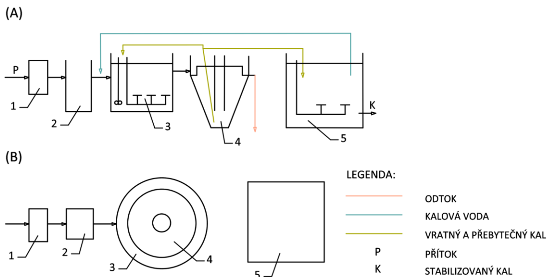
Obr. 4.267: Příklad vzorové technologické linky typizované ČOV: 1 – hrubé předčištění (česle), 2 – vertikální lapák písku, 3 – aktivální nádrž simultánní provoz, 4 – nádrž pro nitrifikaci a denitrifikaci, 5 – vertikální dosazovací nádrž, další objekt mimo schéma – provzdušňovaný kalojem. Schéma Radka Račoch a Michaela Mrvová, 2021 (upraveno dle: poskytnuté projektové dokumentace).
