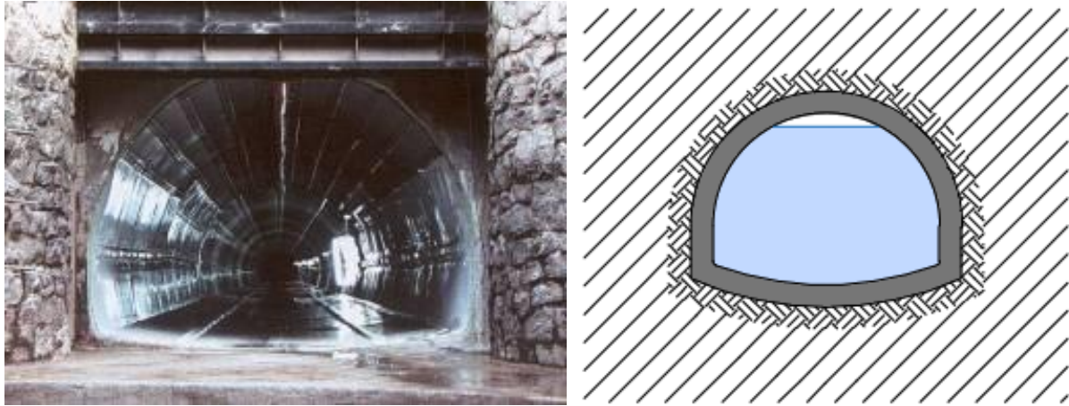
Obr. 4.150: MVE Spálov – štola s volnou hladinou: (A) pohled do štoly po rekonstrukci s použitím geomembrány. Foto převzato z: ZČE, 2000; (B) schéma Radek Míšanec, 2021 (upraveno dle: ZČE, 2000).
