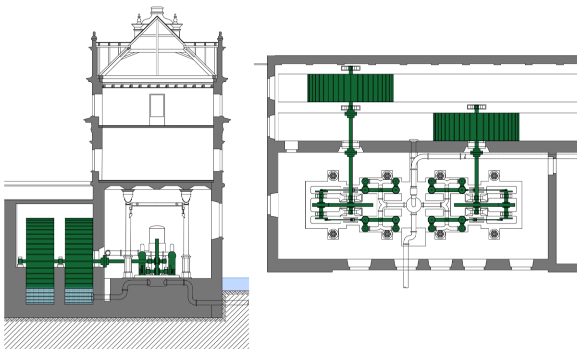
Obr. 4.191: Praha – čerpací stanice Staroměstské vodárny po přestavbě a modernizaci v roce 1882. Stroje z roku 1860 byly nahrazeny čtyřmi dvojčinnými čerpadly Girardova typu, které byly poháněny železnými koly s dřevěnými lopatkami. Schéma Radek Míšanec, 2021 (upraveno dle: plán z APVK, fotoarchiv PVK, kt. N 11, sig. B 013d/88).
