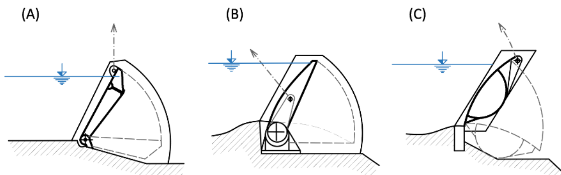
Obr. 4.106: Typy klapkových uzávěrů: (A) Deskové; (B) Troubové; (C) Duté. Schéma Radka Račoch a Michaela Mrvová, 2021 (upraveno dle: Průcha, 1980).
