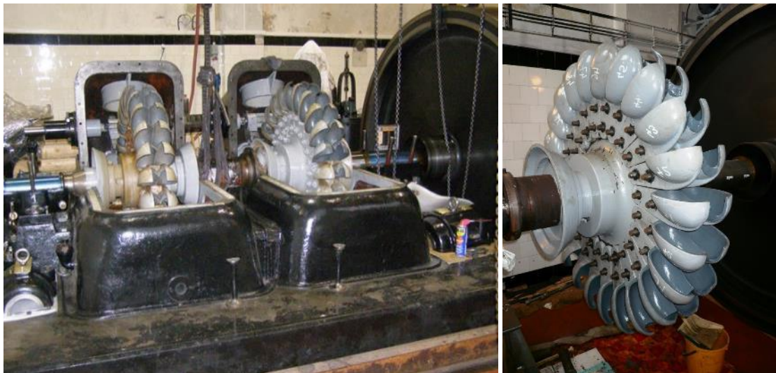
Obr. 4.179: MVE Rudolfov I – dvojčítá horizontální Peltonova turbína v době rekonstrukce. Foto Petr Freiwilg, 2012.
