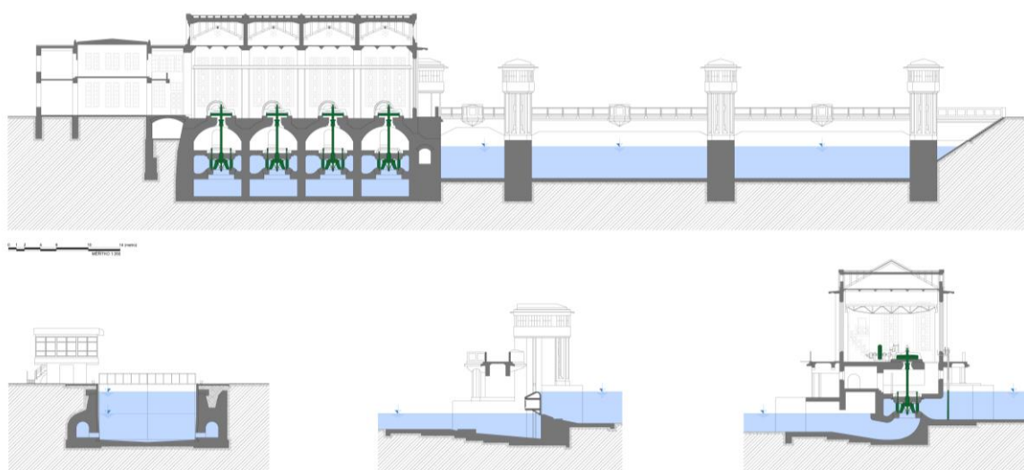
Obr. 4.130: MVE Poděbrady – řezy. Schéma Radek Míšanec, 2018 (upraveno dle: podnikový archiv 1. elektrárenská s.r.o., České Budějovice).
