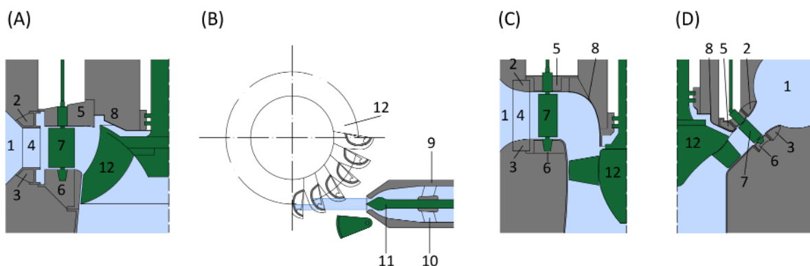
Obr. 4.175: Schémata řešení moderních turbín: (A) Francisova turbína; (B) Peltonova turbína; (C) Kaplanova turbína; (D) Dériezova turbína; 1 – spirála, 2 – horní výztužný kruh, 3 – dolní výztužný kruh, 4 – výztužná lopatka, 5 – horní lopatkový kruh, 6 – dolní lopatkový kruh, 7 – rozváděcí lopatka, 8 – víko turbíny, 9 – dýza, 10 – vodící kříž, 11 – regulační jehla, 12 – oběžné kolo. Schéma Radek Mišanec, 2021 (upraveno dle: Bednář, 1989).
