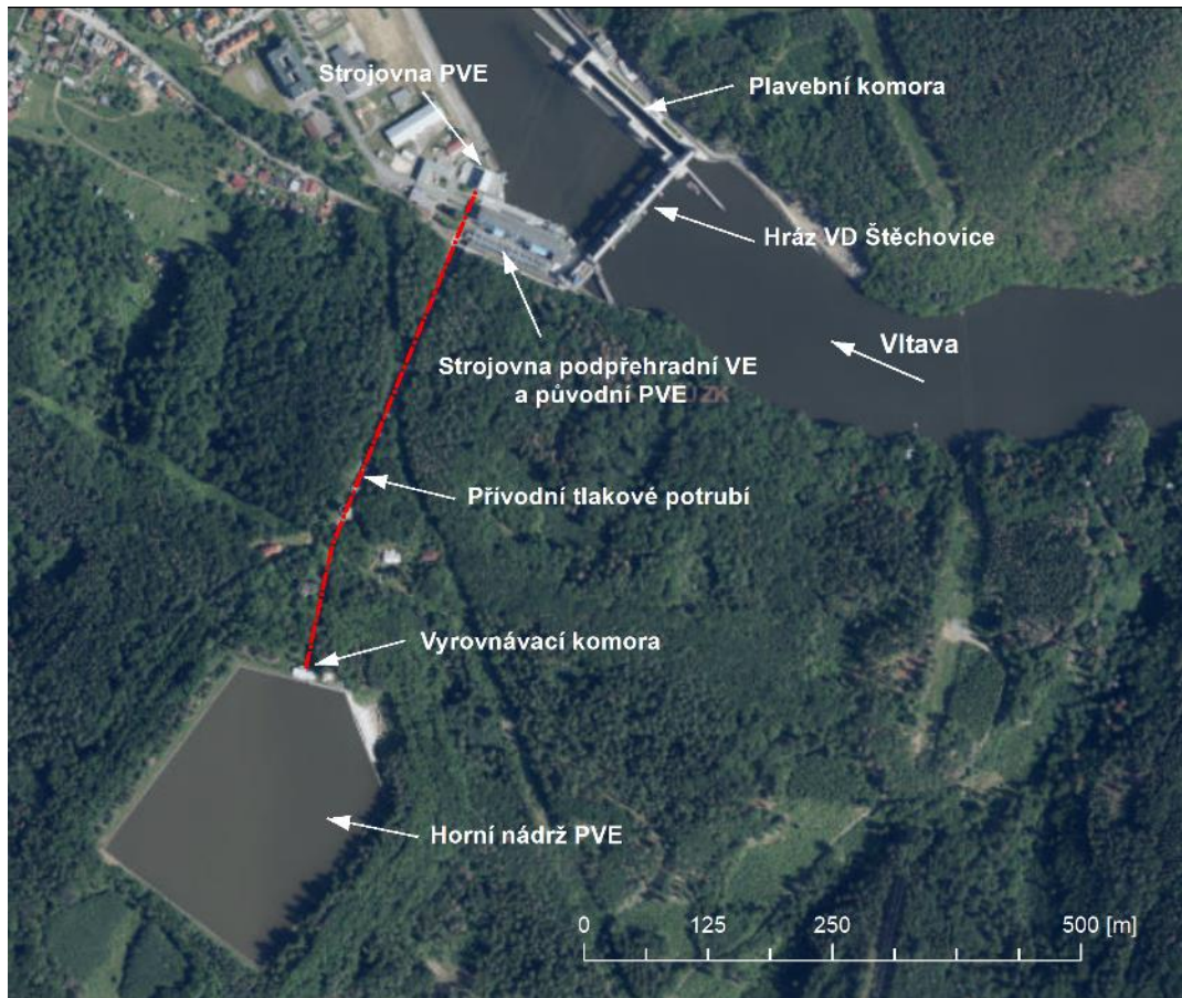
Obr. 4.138: Situace VD Štěchovice s PVE a podpřehradní VE. Situace vytvořena na podkladě dat ČÚZK, 2021.
