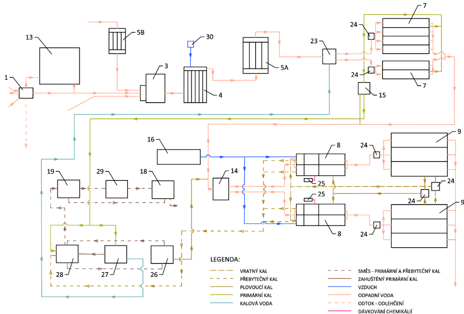
Obr. 4.263: Technologické schéma (linka) brněnské ČOV v současnosti: 1 – rozdělovací objekt na přítoku, 3 – česlovna, 4 – lapák písku, 5A – šneková čerpadárna, 7 – usazovací nádrže, 8 – aktivační nádrže, 9 – dosazovací nádrže, 14 – mezičerpací stanice, 15 – čerpací stanice primárního kalu, 16 – dmychárna, 18 – odvodnění a sušení kalu, 19 – vyhnívací nádrže, 23 – rozdělovací objekt na usazovací nádrže, 24 – šachtice a čerpání, 25 – dávkování chemikálií, 26 – flotační jednotka, 27 – zahušťovací nádrž, 28 – čerpací stanice přepadu flotace. Schéma Radka Račoch a Michaela Mrvová, 2021 (upraveno dle: poskytnuté projektové dokumentace BVaK).
