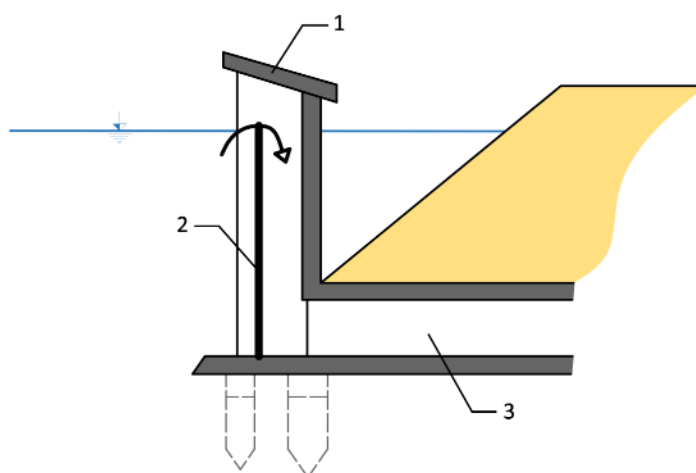
Obr. 4.60: Obecné schéma – otevřený požerák: 1 – koruna požeráku s uzamykatelným poklopem, 2 – dlužová stěna, 3 – potrubí. Schéma Radka Račoch a Radek Bachan, 2021 (upraveno dle: Slavík, Neruda, 2007).
