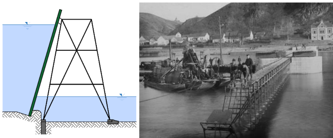
Obr. 4.105: Vlevo hradlový jez. Schéma Radka Račoch a Radek Bachan, 2021 (upraveno dle: Kratochvíl, 1947). Vpravo hradlový jez v Klecanech (převzato z: Klír, 1908.)
