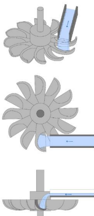
Obr. 4.174: Vodní kolo horizontální. Schéma Radek Míšanec, 2021 (upraveno dle: Zeising, 1612).
