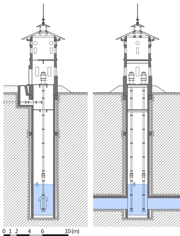
Obr. 4.205: Benešov u Prahy – studna trubní s čerpací stanicí. Schéma Radek Mišanec, 2021 (upraveno dle: Klír a Klokner, 1923).
