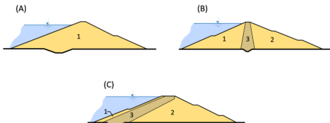
Obr. 4.4: Základní typy zemních přehrad: (A) Zemní homogenní: 1 – část stabilizační; (B) Zemní se středním těsněním: 1 – návodní stabilizační část, 2 – vzdušní stabilizační část, 3 – zemní těsnění (jádro); (C) Zemní s návodním těsněním: 1 – opevnění, 2 – vzdušní stabilizační část, 3 – návodní zemní těsnění. Schéma Radka Račoch, 2021 (upraveno dle: Broža a kol., 2005).
