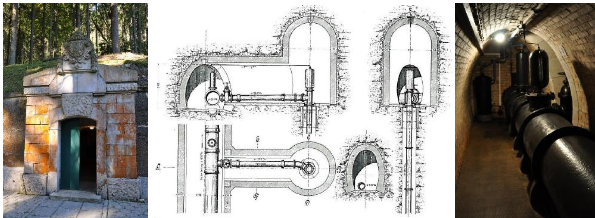
Obr. 4.206: Březová nad Svitavou – vodárenská štola I. březovského vodovodu s násoskovými studnami, původní litinové potrubí z roku 1913, čerpaná voda je gravitačním způsobem vedena do města Brna 56 km dlouhým potrubím. Foto David Honek, 2019, schéma BVK (2013).
