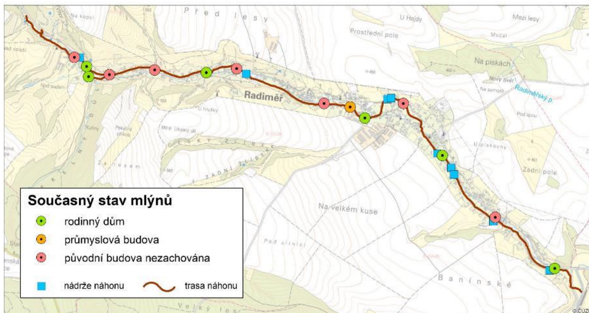
Obr. 3.5: Systém Radiměřského náhonu se 14 mlýny a 9 malými vodními nádržemi – současný stav (trasa náhonu se částečně zachovala jako relikt v terénu); příklad širší soustavy technologického celku, který se skládá z tělesa náhonu včetně ovládacích prvků (stavidla, nátoky na vodní kola), malých vodních nádrží pro zvýšení akumulace vody v náhonu, vodních kol (nedochovaných) se systémovou vazbou na technologie vodních mlýnů, které sami o sobě představují ucelenou fázi technologického toku. Schéma David Honek, 2020.
