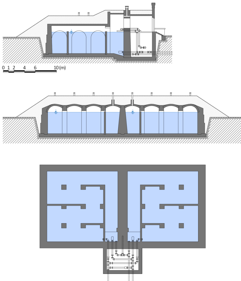
Obr. 4.212: Praha-Vršovice – zemní vodojem Na Zelené Lišce (součást Vršovické vodárny), příklad zemního cihelného vodojemu. Schéma Radek Míšanec, 2021 (upraveno dle: Klír a Klokner, 1923).
