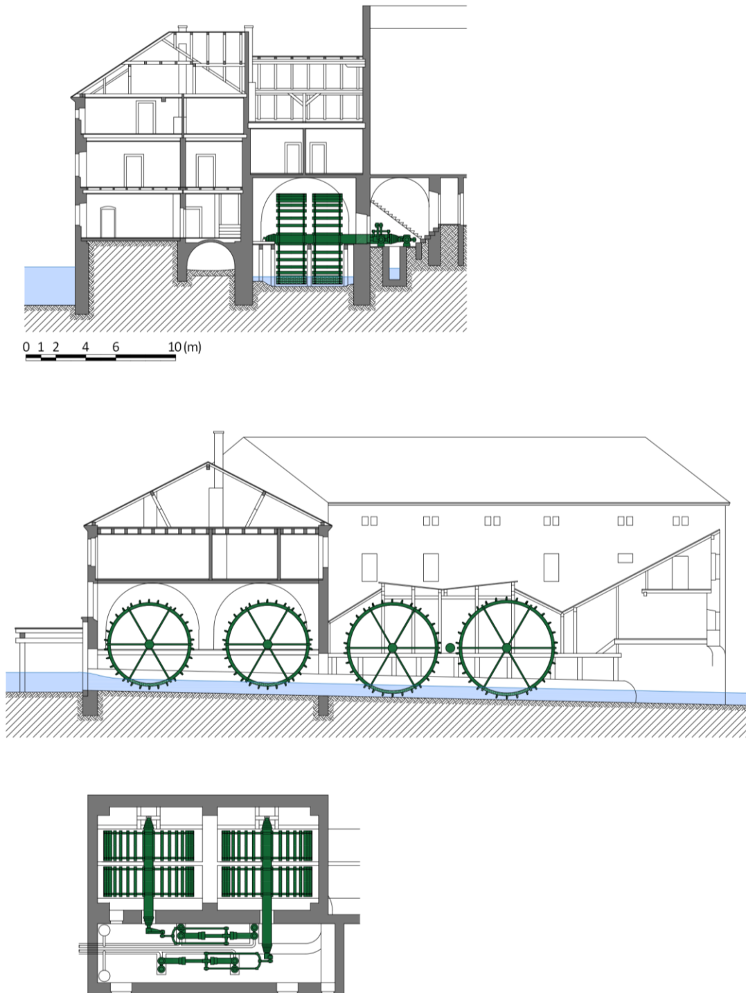
Obr. 4.188: Praha – původní čerpací stanice Staroměstské vodárny (před modernizací v roce 1882), nahoře řez původním objektem a lednicí s původními čtyřmi koly na spodní vodu před jejich demolicí v roce 1882. Točivý pohyb hřídelí vodních kol se převáděl klikou na ojnice jednotlivých pístů čerpacího stroje, který vytlačoval vodu do nádrže v horním patře věže. Původní renesanční čerpací stroj byl vyroben ze dřeva a železa, samotné písty byly vyrobeny z volské kůže a pohybovaly se v mosazných konvích. Tato čerpadla byla vyměněna v roce 1835 a 1860 za nové stroje vyrobené kompletně ze železa. Půdorys zobrazuje pouze jednu polovinu lednice. Schéma Radek Míšanec, 2021 (upraveno dle: plán z APVK, fotoarchiv PVK, kt N 11, sig. B 013a/88).
