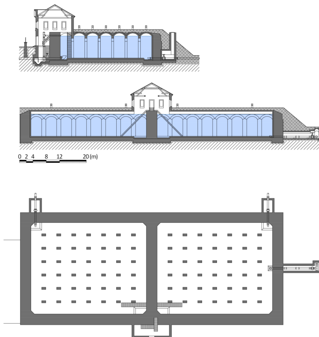
Obr. 4.192: Praha – vodojem na Karlově, kam byla, po jeho vybudování, čerpána voda ze všech funkčních pražských vodáren (Staroměstská, Šítkovská, Novomlýnská, Žofínská, původní Pražská vodárna v Podolí), konkrétně ze Staroměstské vodárny po její rekonstrukci v letech 1882–1884. Schéma Radek Míšanec, 2021 (upraveno dle: plán z APVK, nesignováno).
