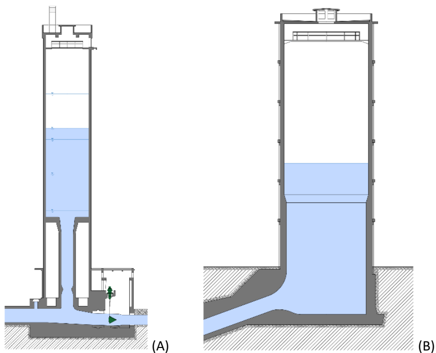
Obr. 4.157: Řez nadzemní vřícovou vyrovnávací komorou s diafragmou: (A) MVE Práčov I; (B) MVE Seč. Schéma Radek Míšanec, 2021 (upraveno dle: Trejtnar, 1975).
