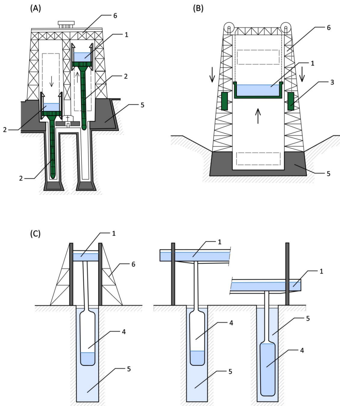
Obr. 4.80: Lodní zdvihadla svislá: (A) Pístové lodní zdvihadlo; (B) Schéma lodního zdvihadla s protizávažím; (C) Schéma plovákového lodního zdvihadla; 1 – nádrž pro přepravu lodě, 2 – hydraulicky ovládaný píst, 3 – protizávaží, 4 – plovák, 5 – pevné technologické prvky, 6 – nadzemní nosné konstrukce. Schéma Radka Račoch, Radek Bachan a Michaela Mrvová, 2021 (upraveno dle: VŠB – TUO, 2013).
