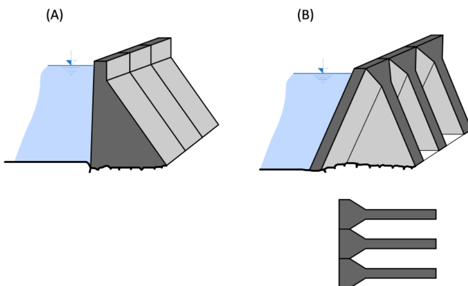
Obr. 4.18: (A) Tízná přehrada; (B) Tízná pilířová přehrada. Schéma Radka Račoch, 2021 (upraveno dle: Broža a kol., 2005).
