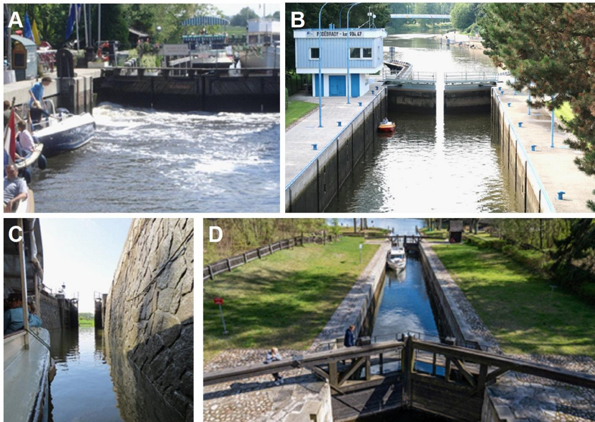
Obr. 4.79: Příklad plavebních komor: (A) Holandsko, napouštění komory obtokem vrat; foto V. Forejtník, 2007; (B) Poděbrady, komora s ocelovými vraty plnicími otvory obtokových kanálů; foto Miriam Dzuráková, 2021; (C) Zdymadlo na Batově kanálu na dolní vodě, kyklopské zdivo; archiv VÚV, 2012; (D) – Polsko, zdymadlo s dřevěnými vraty na Augustovském kanálu; foto osobní archiv Mileny Forejtníkové.
