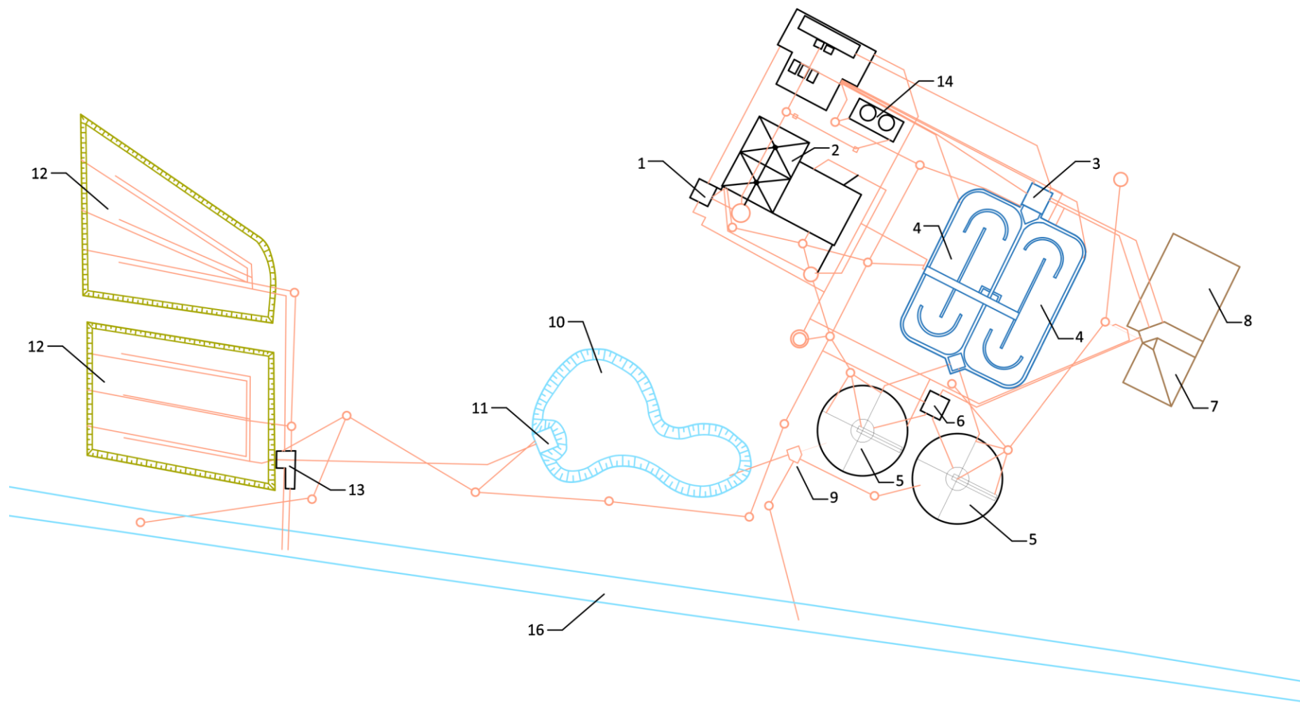
Obr. 4.266: Technologické schéma (linka) ČOV pro větší obec do 10 tisíc obyvatel (Harmannsdorf, Rakousko): 1 – přítok, čerpací stanice, 2 – provozní budova, 3 – selektor (rozdělovač vody), 4 – oběhová aktivace, 5 – dosazovací nádrže, 6 – čerpadlo na kal, 7 – zpracování kalu (odvodnění), 8 – prostor uložení kalu, 10 – dočišťovací stabilizační nádrž rybníčního typu, 11 – odtokový biofiltr, 12 – kořenová čistírna, 13 – kontrolní a měřící šachtice, 14 – biofiltr na čištění vzduchu z prostoru ČOV, 15 – studna, 16 – recipient vyčištěných vod (místní vodní tok). Schéma Radka Račoch a Michaela Mrvová, 2021 (upraveno dle: poskytnuté projektové dokumentace).
