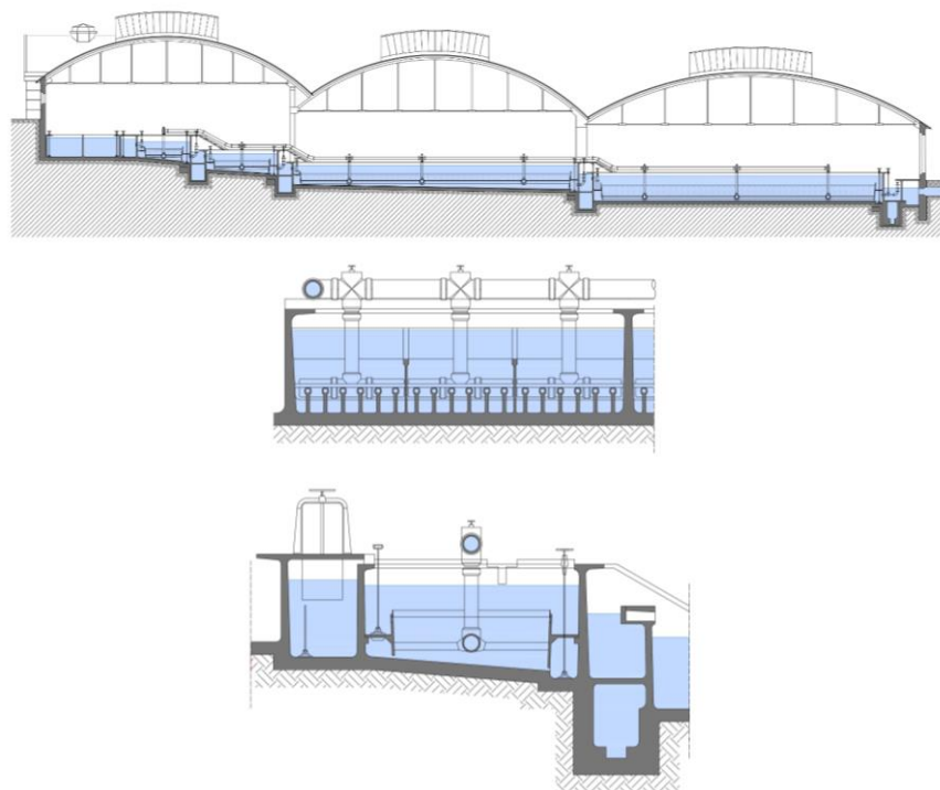
Obr. 4.210: Plzeň – městská říční vodárna v Malostranské ulici na Homolce, filtrační stanice systému Puech-Chabal o celkové ploše filtrace 5 000 m 2 se třemi stupni hrubocozů s tzv. horním praním a jedním stupněm
