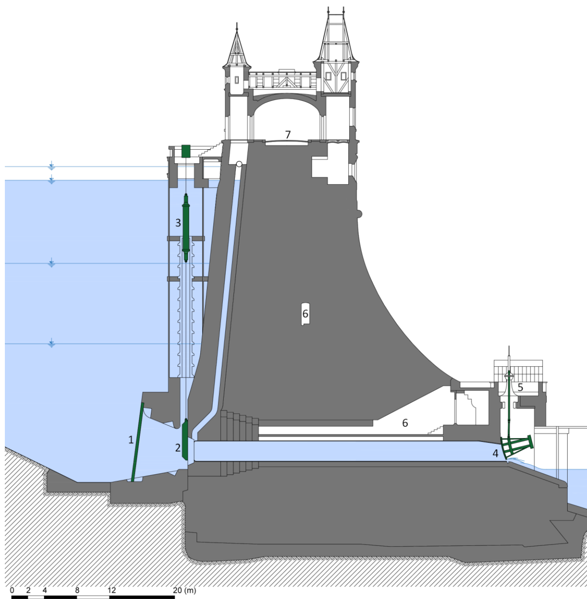
Obr. 4.40: Přehrada Les Království (1910–1919) – příčný řez hrází v místě spodní výpusti: 1 – česle, 2 – tabulový uzávěr, 3 – ovládání tabulového uzávěru, 4 – segmentový uzávěr, 5 – ovládání segmentového uzávěru, 6 – revizní štola, 7 – koruna hráze. Schéma Radek Míšanec, 2021 (upraveno dle: archiv Povodí Labe).
