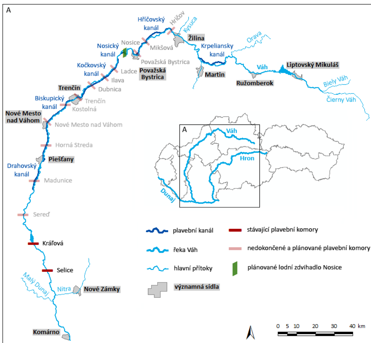
Obr. 4.118: Vážská kaskáda a vodní cesta. Schéma Radek Bachan, 2021.
