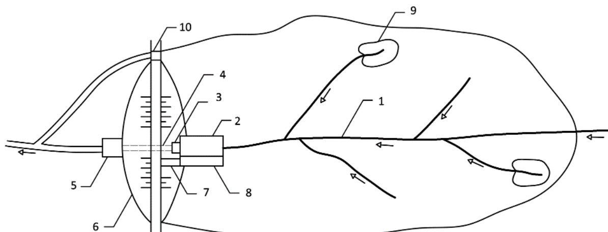
Obr. 4.69: Schéma rybochovné nádrže s objekty a speciálně upraveným dnem: 1 – hlavní odvodová stoka, 2 – loviště, 3 – požerák, 4 – potrubí, 5 – vývařiště, 6 – hráz, 7 – přístupové schody, 8 – kádiště, 9 – odvodnění prohlubní, 10 – bezpečnostní přeliv. Schéma Radka Račoch a Radek Bachan, 2021 (upraveno dle: Pokorný, 2009).
