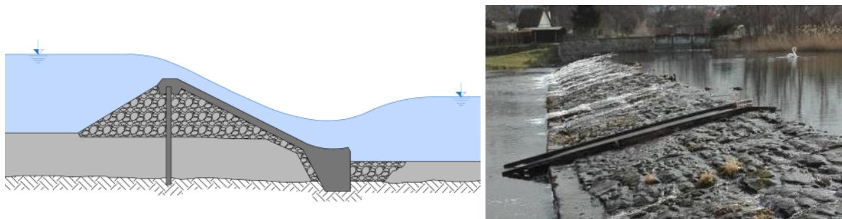
Obr. 4.100: Vlevo kamenný jez. Schéma Radek Míšanec, 2021 (upraveno dle: Gabriel a kol., 1989); Vpravo jez u Oblekovic (převzato z: PMO, 2019a).
