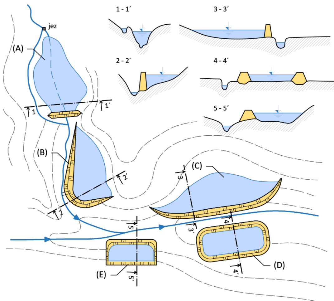
Obr. 4.47: Typy neprůtočných nádrží a jejich průřezy: (A) – údolní obtoková, (B) – břehová, (C) – boční, (D) – hrázová, (E) – kopaná. Schéma Radka Račoch a Radek Bachan, 2021 (upraveno dle: Šálek, 1996).
