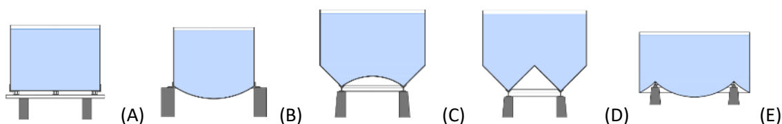
Obr. 4.218: Příklady dna kovových nádrží: (A) rovné dno; (B) dno ve tvaru kulového vrchlíku vypouklého dolů nebo nahoru, Barkhausen; (C) a (D) dno s vnějším pláštěm kuželovým a vnitřním ve tvaru kulového vrchlíku nebo kuželovým, prof. Inze; (E) dno složené z vnitřního visutého vrchlíku a vnějšího visutého pláště kuželového, Smreker. Realizace posledních dvou typů (D) a (E) nejsou v ČR doloženy. Schéma Radek Míšanec, 2021 (upraveno dle: Klír a Klokner, 1923 a archivní plánové dokumentace).
