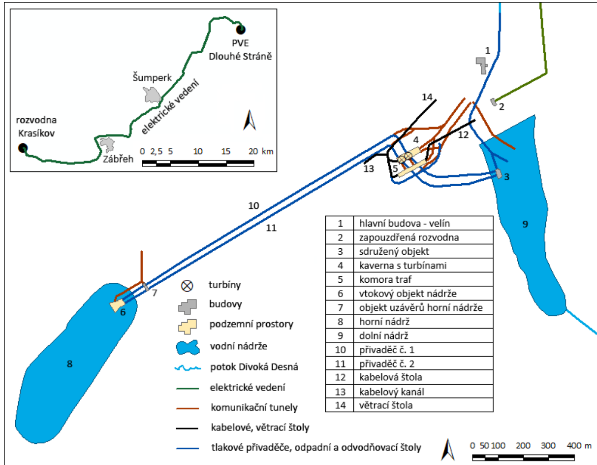
Obr. 4.184: PVE Dlouhé Stráně – přehledová mapa, včetně vedení velmi vysokého napětí. Schéma Radek Bachan, 2021 (upraveno dle: Kopřiva a kol. 1997; ZAO – SOkA Šumperk, PVE Dlouhé Stráně – Souhrnné řešení stavby; RUIAN; ZABAGED).
