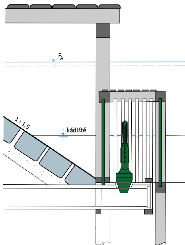
Obr. 4.58: Čepový uzávěr: F_A – maximální hladina. Schéma Radka Račoch a Michaela Mrvová, 2021 (upraveno dle: Pavelková a kol., 2014).
