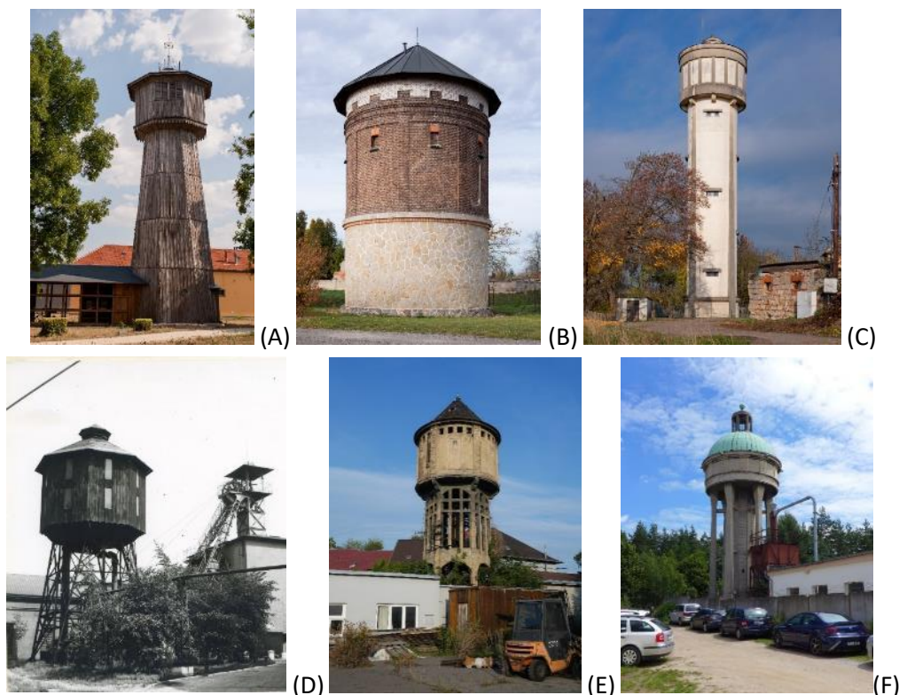
Obr. 4.217: Příklady nosných konstrukcí věžových vodojemů: (A) Palárikovo (Slovensko), dřevěný věžový vodojem, zřejmě jediný zachovalý v Evropě, po konverzi. Foto ARCHINFO (2015); (B) Kovanec, věžový vodojem se stěnovou nosnou konstrukcí zděnou z kamene a cihelného zdiva, postavený v historizujícím tvarosloví podle návrhu Karla Kresse v roce 1909. Foto Viktor Mácha, 2018; (C) Horní Bukovina, věžový vodojem se železobetonovou nosnou konstrukcí postavený roku 1935 podle návrhu Ing. Fanty. Foto Viktor Mácha, 2018; (D) Ostrava, důl Hubert, zaniklý věžový vodojem s ocelovou nosnou skeletovou (příhradovou) konstrukcí a dřevěným opláštěním nádrže na snímku z konce 60. let 20. století. Foto reprofoto archiv MCPD; (E) Duchcov, věžový vodojem se skeletovou železobetonovou nosnou konstrukcí postavený v letech 1908–1912 pro sklárnu Engels. Foto Michaela Ryšková, 2020; (F) Lázně Bohdaneč, věžový vodojem nesený železobetonovou kombinovanou konstrukcí, postavený podle návrhu Josefa Gočára v roce 1911, ve středním dříku konstrukce je umístěno schodiště. Foto Michaela Ryšková, 2016.
