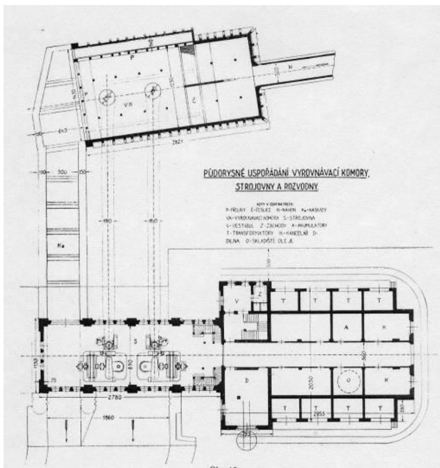
Obr. 4.156: Dispoziční uspořádání vyrovnávací komory, přívodního tlakového potrubí a strojovny MVE Spálov (převzato z: ZSV, 1924)
