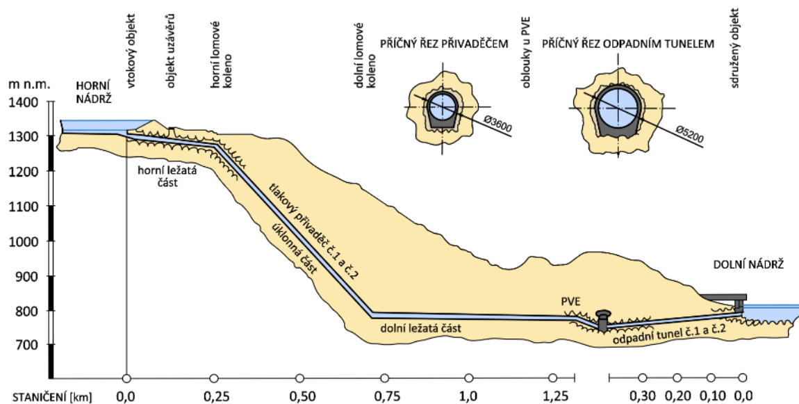
Obr. 4.185: PVE Dlouhé Stráně – schéma hydraulického obvodu. Schéma Radka Račoch a Michaela Mrvová, 2021 (upraveno podle: Kopřiva a kol., 1997).
