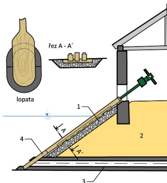
Obr. 4.59: Lopatový uzávěr: 1 – kamenný zához, 2 – těleso hráze, 3 – spodní výpust, 4 – spodní část lopaty. Schéma Radka Račoch a Michaela Mrvová, 2021 (upraveno dle: Vrána, Beran, 2008).
