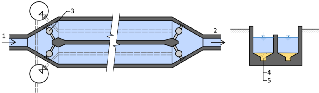
Obr. 4.240: Komorový lapák písku: 1 – přítok, 2 – odtok, 3 – stavidlo, 4 – filtrační materiál, 5 – drenáž. Schéma Radka Račoch a Radek Bachan, 2021 (upraveno dle: archiv VÚV).
