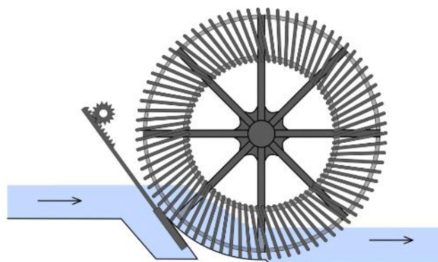
Obr. 4.171: Vodní kolo Sagebienovo. Schéma Radka Račoch a Michaela Mrvová, 2021 (upraveno dle: Hýbl 1922; Štěpán a kol. 2008; Štěpán, 1990; Digitalisierung des Polytechnischen Journals, 2021).
