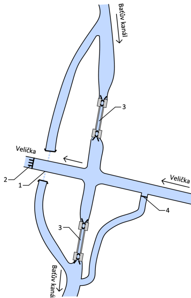
Obr. 4.86: Schéma křížení Baťova kanálu a Veličky: 1 – shybka pro udržení stejné hladiny plavebního kanálu, 2 – jez upravující hladinu Veličky, 3 – plavební komory se zdvojenými vraty, 4 – stavidlo. Schéma Radka Račoch a Radek Bachan, 2021 (upraveno dle situace v terénu 2020).
