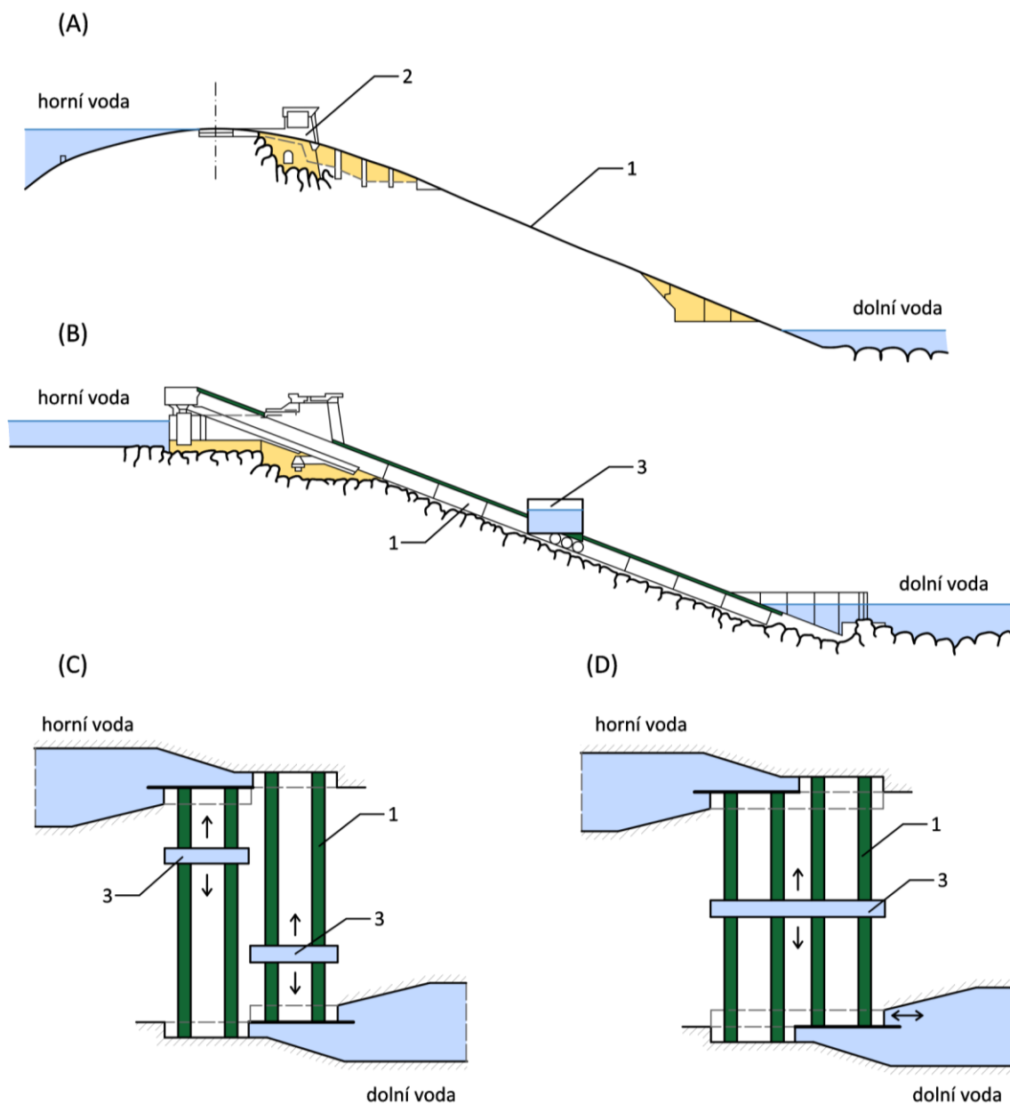
Obr. 4.81: Lodní zdvihadla šikmá – výtahy: (A) Kolejová přeprava menších lodí na vozíku; (B) kolejová přeprava větších plavidel v přímém pohyblivém žlabu; (C) Příčný pohyblivý žlab, zdvojená kolejová dráha; (D) Možnost spojení dvou žlabů pro přepravu dlouhých člunů; 1 – kolejová dráha, 2 – vozík pro přepravu malých lodí, 3 – pohyblivý žlab pro přepravu větších plavidel. Schéma Radka Račoch, Radek Bachan a Michaela Mrvová, 2021 (upraveno dle: Březinský, 2020 a VŠB – TUO, 2013)
