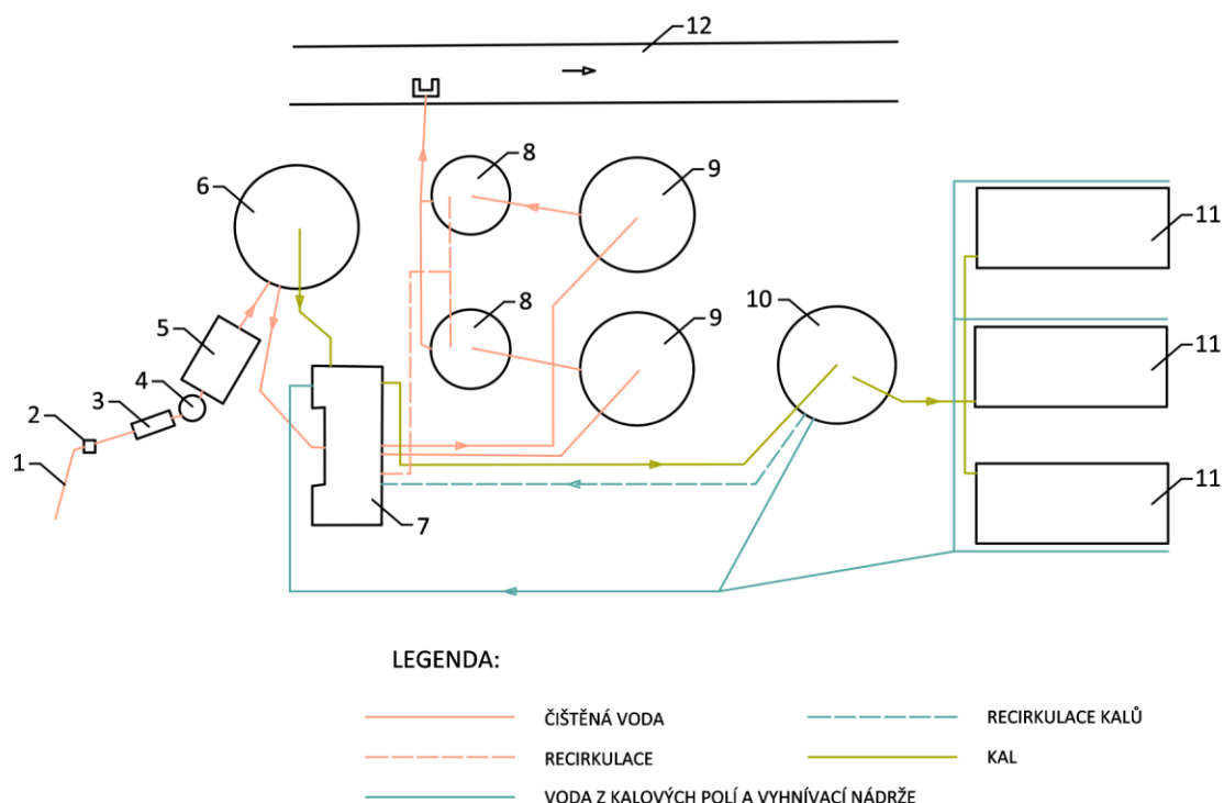
Obr. 4.264: Technologické schéma (linka) ČOV Kuřim: 1- Přítok surové vody, 2 – vypínací šachta, 3 – česle, 4 – lapák písku, 5 – lapák tuku, 6 – usazovací nádrž typu DORR, 7 – strojovna, 8 – dosazovací nádrže, 9 – skrápěné biofiltry, 10 – vyhnívací komora na kal, 11 – kalová pole, 12 – recipient vyčištěných odpadních vod (místní vodní tok). Schéma Radka Račoch a Michaela Mrvová, 2021 (upraveno dle: poskytnuté projektové dokumentace BVaK).
