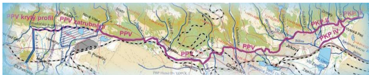
Obr. 4.96: Podkrušnohorský přivaděč. Schéma z materiálů podniku Povodí Ohře vydaných pro veřejnost.
