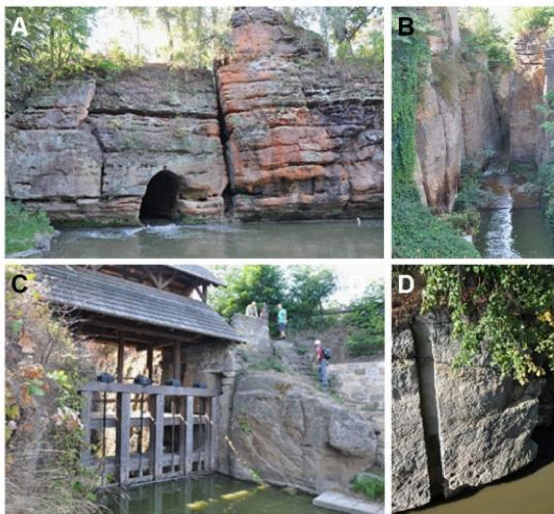
Obr. 4.90: Stavební materiál vodních kanálů - pískovec: (A) a (B) Průrva Ploučnice, umělé zkrácení toku tunelem a otevřeným korytem; (C) osazení objektu se stavidly přímo do pískovcového skalního bloku; (D) detail drážky pro provizorní hrazení vysekaný v pískovci. Foto David Honek, 2019
