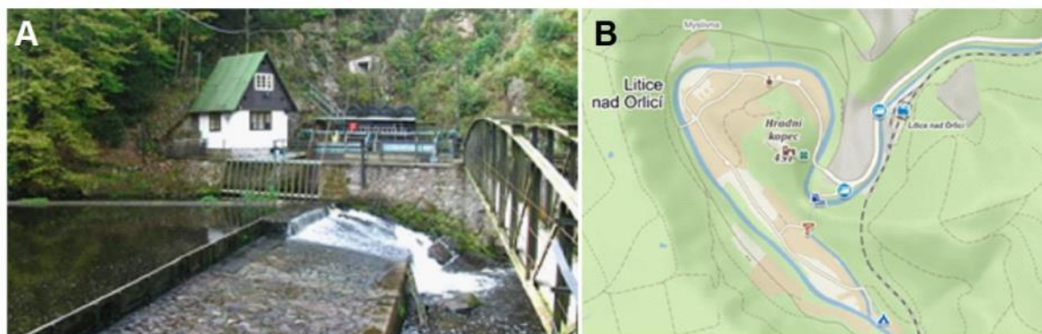
Obr. 4.88: Litice nad Orlicí: (A) jez s nátokem do průpichu. Foto Milena Forejtníková, 2020; (B) Situace lokality v mapě (převzato z: mapy.cz).
