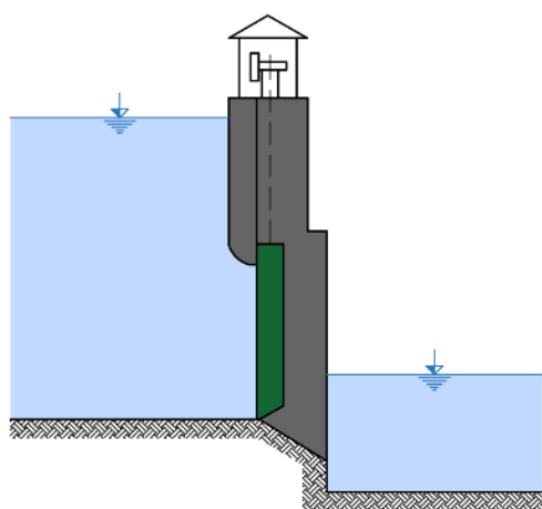
Obr. 4.108: Vlevo stavidlový (tabulový) jez zdvižný. Schéma Radka Račoch a Radek Bachan, 2021 (upraveno dle: Gabriel a kol., 1989). Vpravo stavidlový jez na Metuji v Hronově (převzato z: vodnimlyny.cz, 2013.)
