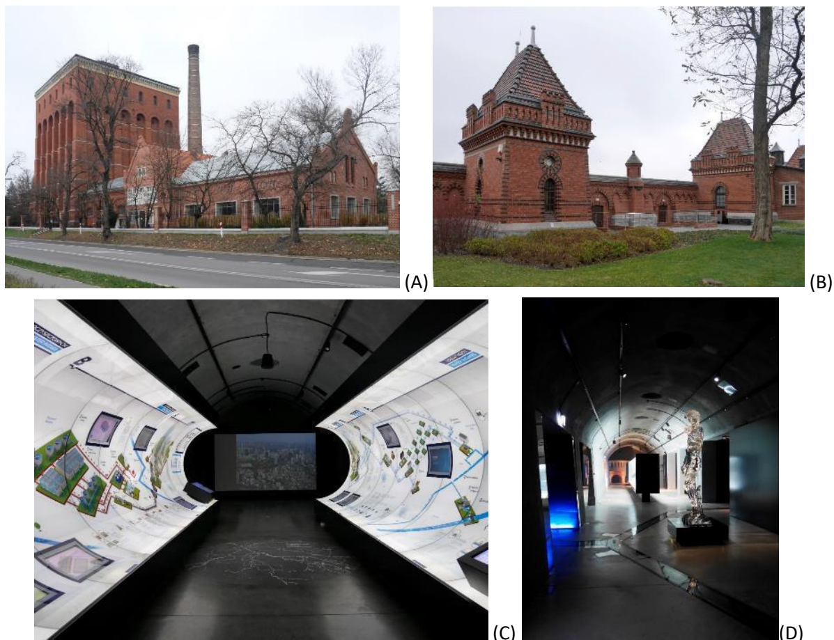
Obr. 5.17: Vratislav (Polsko) – čerpací stanice a zemní vodojem Na Grobli: (A) věžový vodojem a parní čerpací stanice dochovaná včetně původního vybavení, veřejnosti nepřístupná; (B) zemní vodojem; (C) a (D) současná expozice Hydropolis v bývalém zemním vodojemu. Foto Michaela Ryšková, 2019.
