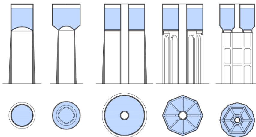
Obr. 4.216: Příklady konstrukčního řešení vodojemů se železobetonovou konstrukcí. Schéma Radek Míšanec, 2021 (upraveno dle: Klír a Klokner, 1923).
