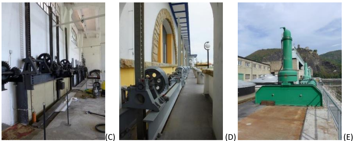
Obr. 4.139: Stavidlové uzávěry a čistící stroje na vtcích jezových MVE: (A) a (D) MVE Miřejevice. Foto VUT v Brně, FAST, 2014; (B) MVE Kroměříž. Foto Miloš Matěj, 2016); (C) MVE Háj – Třeština. Foto Michaela Ryšková, 2018; (E) VE Střekov. Foto Michaela Ryšková, 2015.
