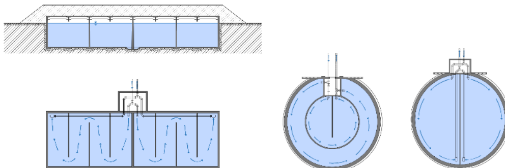
Obr. 4.211: Čtverhranný a kruhový zemní vodojem. Schéma Radek Míšanec, 2021 (upraveno dle: Klír a Klokner, 1923).
