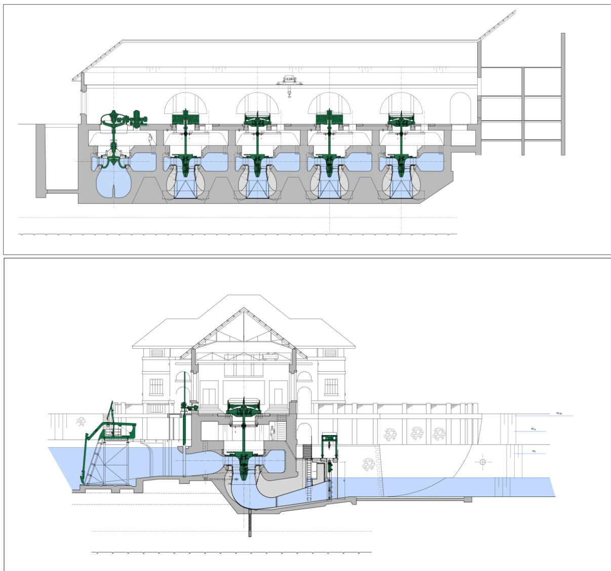
Obr. 4.126: MVE Miřejovice na krátkém přivaděči – řezy (převzato z: Aquatis, a.s.).
