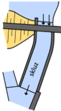
Obr. 4.27: Postranní bezpečnostní přeliv. Schéma Radka Račoch a Radek Bachan, 2021 (upraveno dle: Broža a kol., 1987).
