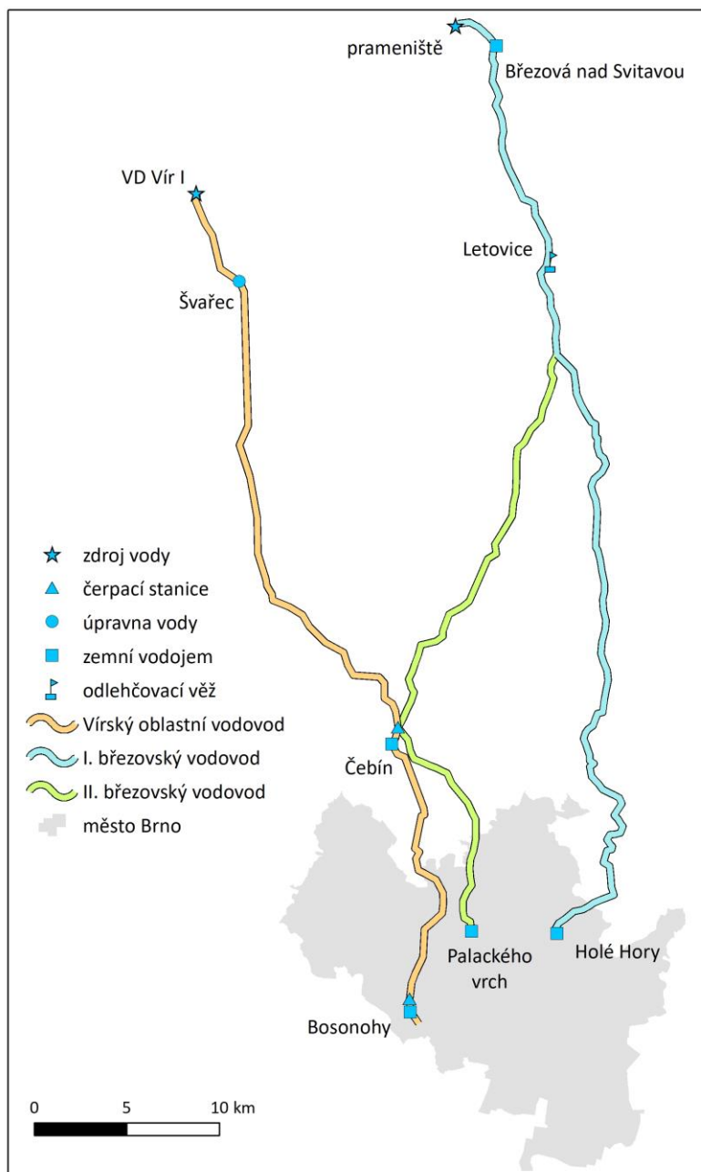
Obr. 4.230: Zásobování města Brna. Schéma David Honek, 2021.
