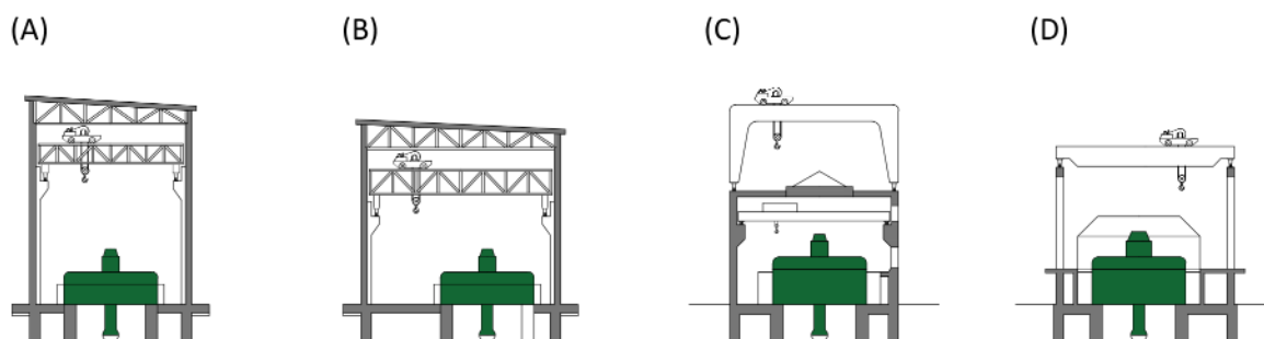
Obr. 4.158: Typy uspořádání horní stavby strojovny: (A) a (B) zakrytá; (C) polozakrytá; (D) odkrytá – bez horní stavby. Schéma Radek Míšanec, 2021 (upraveno dle: Hodák, 1998).
