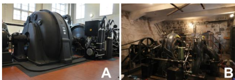
Obr. 5.7: MVE Rudolfov – interiér strojovny: (A) MVE Rudolfov I s Peltonovou turbínou; (B) MVE Rudolfov II s Francisovou turbínou. Foto Petr Freiwillich, 2014 (A), 2013 (B).
