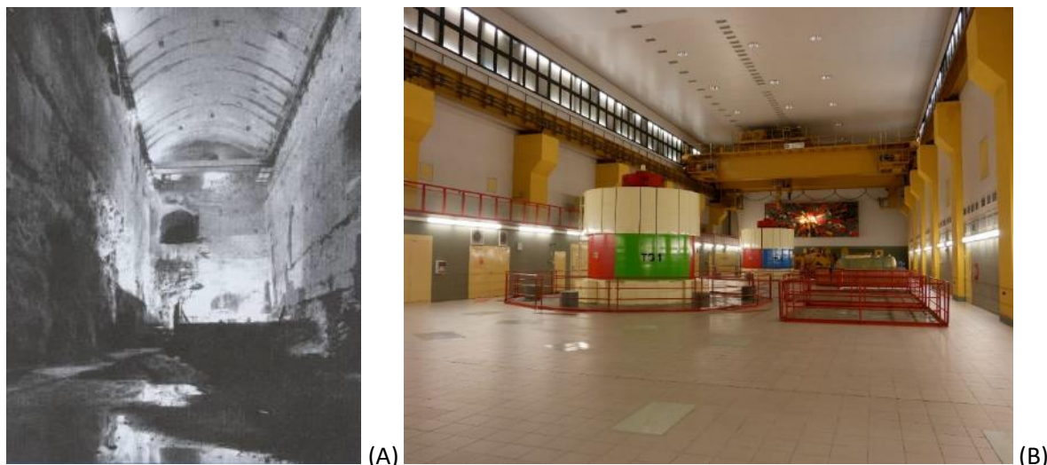
Obr. 4.163: PVE Dlouhé Stráně – podzemní strojovna: (A) kaverna strojovny během výstavby (převzato z: Höll, 1997); (B) současný stav strojovny. Foto Michaela Ryšková, 2019.
