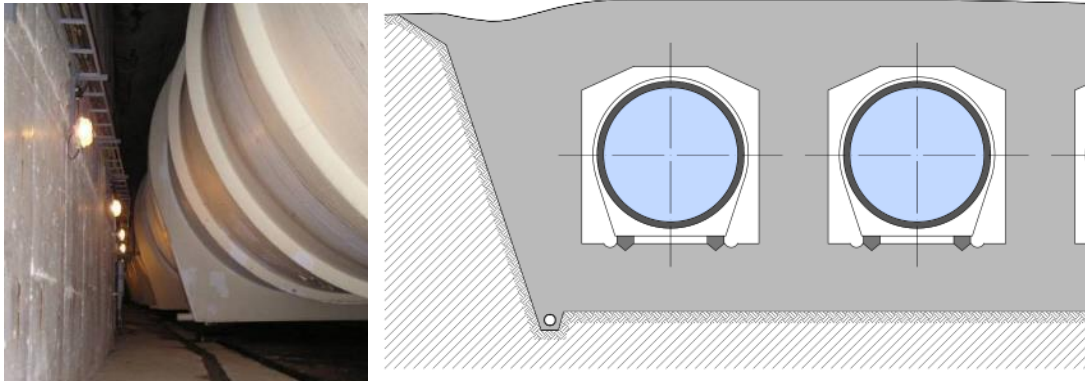
Obr. 4.153: PVE Dalešice – tlakové turbínové ocelové potrubí uložené v chodbě. Foto VUT v Brně, FAST, 2015. Schéma Radek Míšanec, 2021 (upraveno dle: Hynková, 1984).
