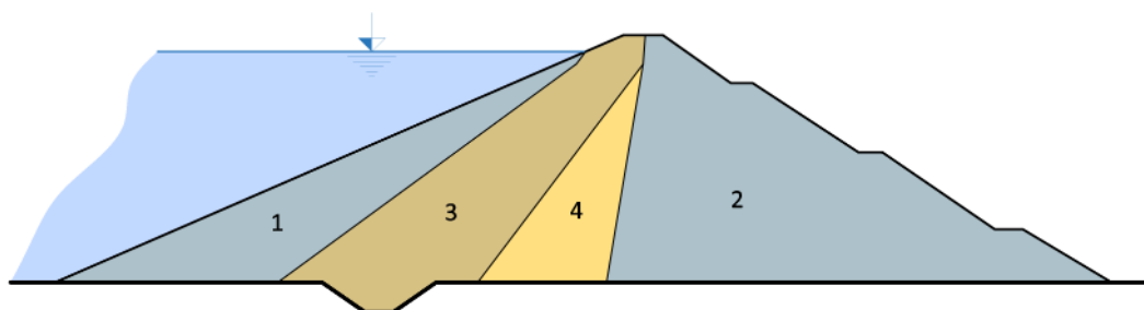
Obr. 4.6: Zonální přehrada: 1 – návodní stabilizační část z lomového kamene, 2 – vzdušná stabilizační část z lomového kamene, 3 – zemní těsnění, 4 – vzdušná stabilizační část ze zeminy. Schéma Radka Račoch, 2021 (upraveno dle: Broža a kol., 2005).
