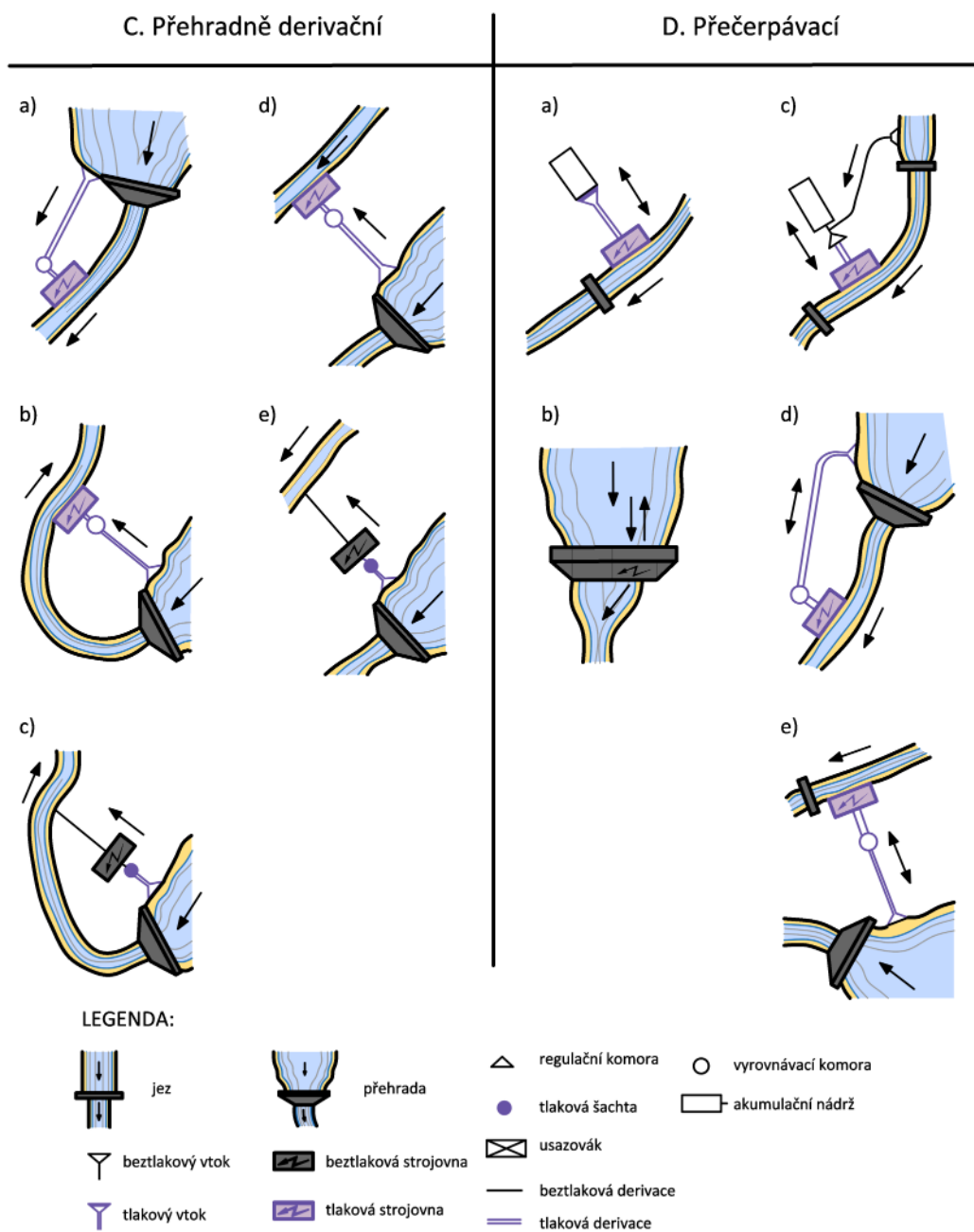
Obr. 4.124: Přehradně derivační a přečerpávací schémata hydroenergetických děl. Schéma Radka Račoch a Michaela Mrvová, 2021 (upraveno dle: Broža a kol., 1990, Čábelka, 1958).
