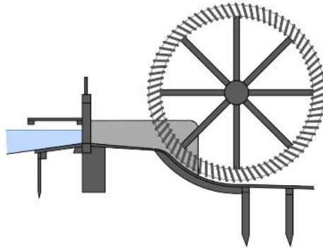
Obr. 4.169: Vodní kolo na spodní vodu s voletem. Schéma Radka Račoch a Michaela Mrvová, 2021 (upraveno dle: Neumann, 1862).
