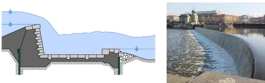
Obr. 4.101: Vlevo zděný jez. Schéma Radka Račoch a Radek Bachan, 2021 (upraveno dle: Průcha, 1980). Vpravo Helmovský jez na Vltavě (převzato z: raft.cz, 2021).
