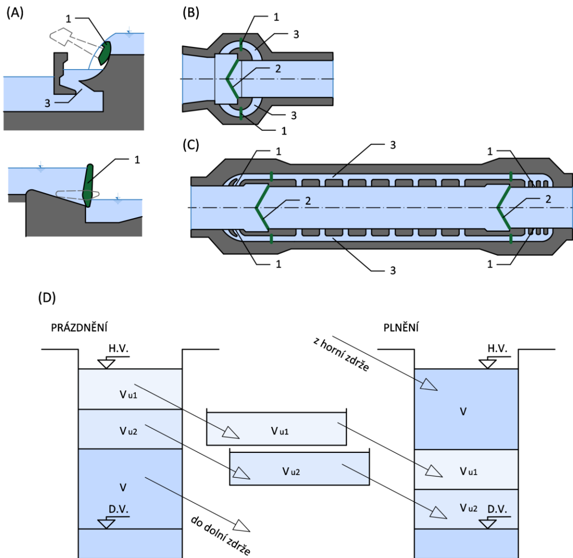
Obr. 4.78: Schéma plnění a prázdnění plavební komory: (A) Plnění vraty; (B) Plnění obtoky u vrat; (C) S plnicími otvory po celé délce komory; 1 – uzávěr náпустných otvorů, 2 - vrata plavební komory, 3 – nátokové a obtokové otvory; (D) Plavební komora s úspornými nádržemi. Schéma Radka Račoch a Radek Bachan, 2021 ((A) – (C) upraveno dle: VŠB – TUO, 2013, (D) dle Moravová, 2020).
