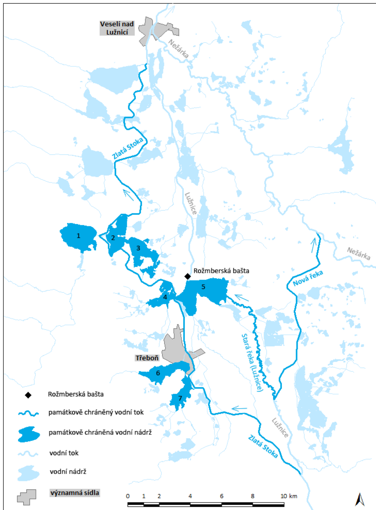
Obr. 4.71 Schéma KP Rožmberská rybníční soustava: 1 – Dvořiště, 2 – Koclířov, 3 – Velký Tisý, 4 – Káňov, 5 – Rožmberk, 6 – Svět, 7 – Opatovický rybník. Schéma Radek Bachan, 2021.
