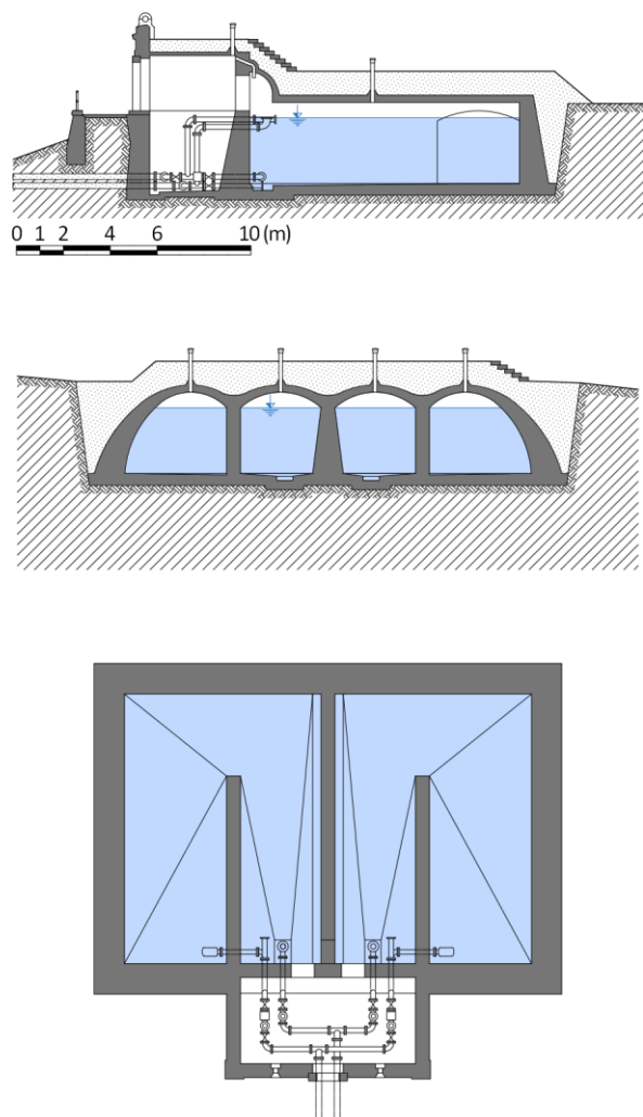
Obr. 4.213: Jičín – zemní vodojem betonový obdélníkového půdorysu. Schéma Radek Míšanec, 2021 (upraveno dle: Klír a Klokner, 1923).
