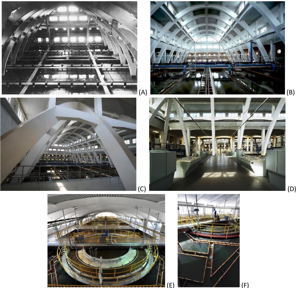
Obr. 4.233: Úpravna vody Praha-Podolí: (A) původní hala filtrace ve 30. letech; (B) současné filtrační nádrže; (C) a (D) pohled na podpěrný obloukový systém; (E) a (F) jedna z hal čiřičů. Foto Archiv PVK a Jaroslav Beneš, 2018.
