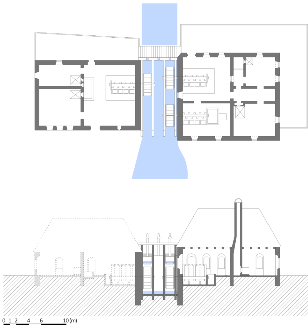
Obr. 4.181: Brno-Husovice – soukenická valcha, rekonstrukce stavu na konci 18. století. Schéma Radek Míšanec, 2018 (dle: Freudenberger, 1977).
