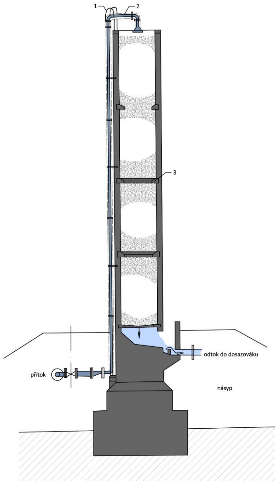
Obr. 4.247: Věžový biofiltr: 1 – ocelový žebřík, 2 – tepelně izolované potrubí pro přívod čišťené vody, 3 – odrazník, uvnitř konstrukce – filtrační náplň (písek, štěrk, směs různých frakcí). Schéma Radka Račoch a Michaela Mrvová, 2021.
