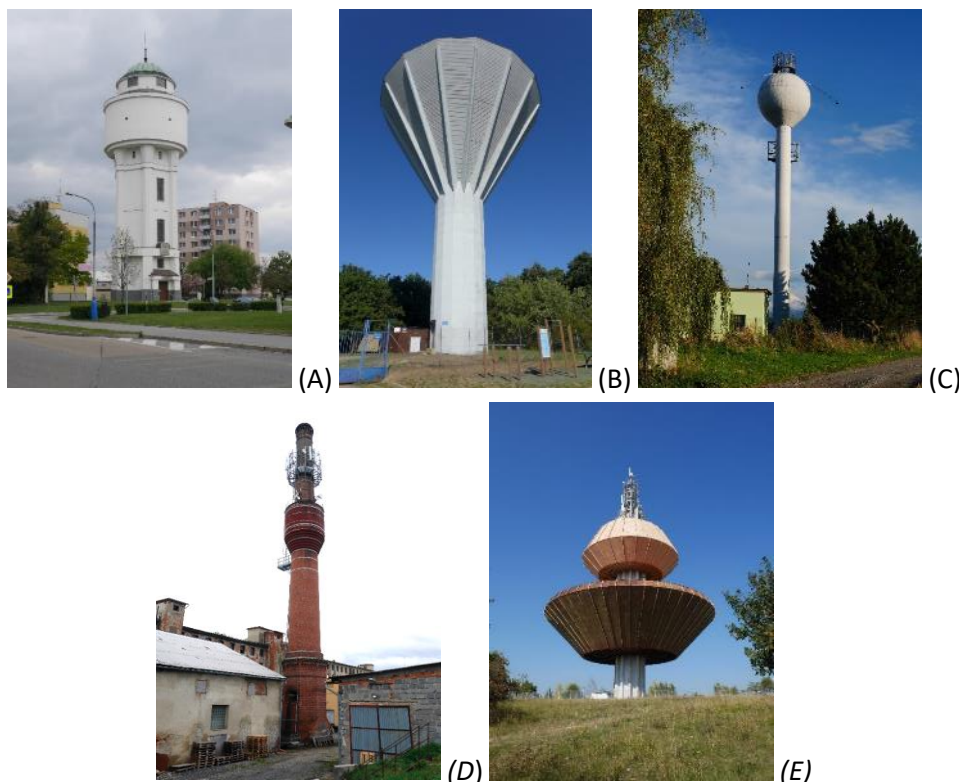
Obr. 4.219: Příklady nádrží věžových vodojemů: (A) Břeclav, železobetonový věžový vodojem z let 1926–1927 s válcovou nádrží nesenou sedmi betonovými dříky. Foto Michaela Ryšková, 2017; (B) Brno-Kohoutovice, věžový vodojem s kuželovou nádrží, realizovaný v roce 1969 dle projektu architekta Tomáše Černouška; první věžový vodojem obdobného typu a konstrukce Svampen byl postaven v roce 1958 ve švédském Örebro. Foto Michaela Ryšková, 2016; (C) Petřvald, věžový vodojem s kulovitou nádrží. Foto Michaela Ryšková, 2021; (D) Sudkov, ocelový válcový komínový vodojem s kuželovým dnem, postavený pro hasební účely v přádelně Inu a bavlny Ig. Seidl v roce 1907. Foto Michaela Ryšková, 2019; (E) Teplice, věžový vodojem se dvěma kovovými nádržemi kombinujícími tvary komolých kuželů. Foto Michaela Ryšková, 2020.
