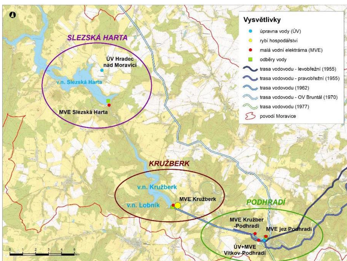
Obr. 3.4: Ostravský oblastní vodovod (Opavská větev) – příklad širší soustavy technologického celku; tento celek lze rozdělit na tři hlavní funkční celky, které jsou vzájemně propojené; jednotlivé funkční celky obsahují objekty, které samy o sobě představují ucelené fáze technologického toku nebo celý technologický tok (přehrada s MVE, úprava vody, dálkový přivaděč vody, jez s MVE). Schéma David Honek, 2021.
