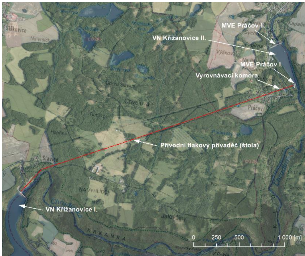
Obr. 4.137: Situace přehradně-derivační MVE Práčov I. a podpřehradní MVE Práčov II. Situace vytvořena na podkladě dat ČÚZK, 2021.
