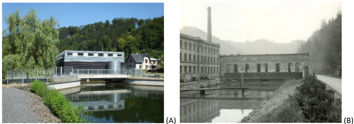
Obr. 4.135: MVE Železný Brod: (A) aktuální strojovna v novém umístění. Foto VUT v Brně, FAST, 2020; (B) původní strojovna v roce 1965. Archiv společnosti Vodní elektrárna Železný Brod, a.s.
