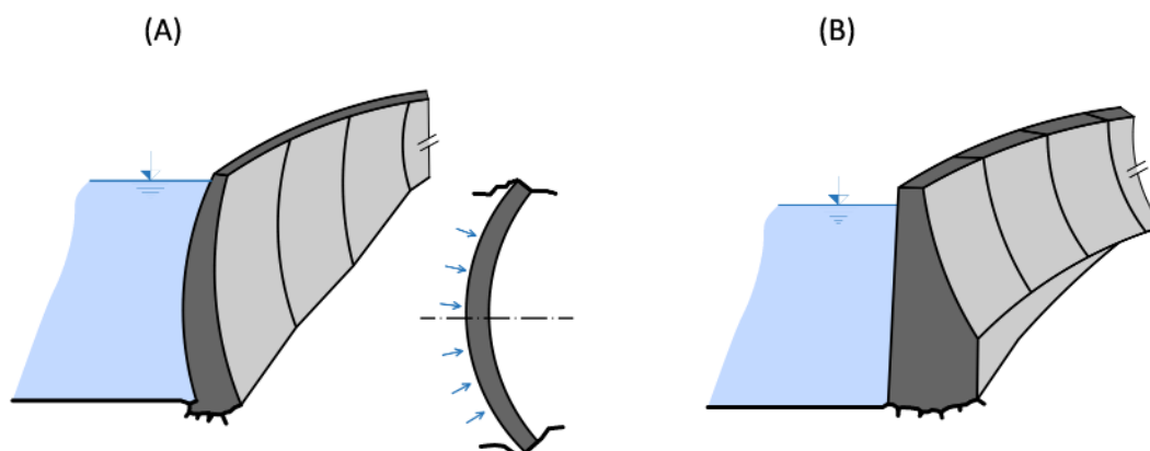
Obr. 4.20: (A) Klenbová přehrada; (B) Klenbová přehrada s tížným účinkem. Schéma Radka Račoch, 2021 (upraveno dle: Broža a kol., 2005).
