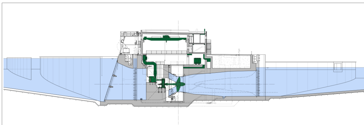
Obr. 4.127: MVE Litoměřice – podélný řez (převzato z: Aquatis, a.s.).
