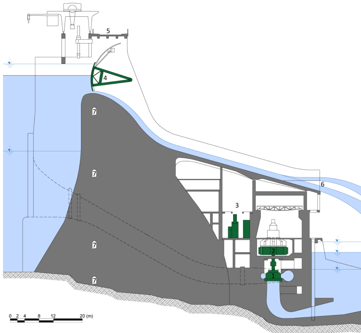
Obr. 4.133: Přehradní podpřepadová VE Slapy: 1 – Kaplanova turbína, 2 – generátor, 3 – rozvodna, 4 – segmentový uzávěr bezpečnostního přelivu, 5 – mostovka, 6 – zakončení skluzu s rozrážeči, 7 – tížná betonová hráz. Schéma Radek Míšanec, 2021 (upraveno dle: Štoll, 1977).
