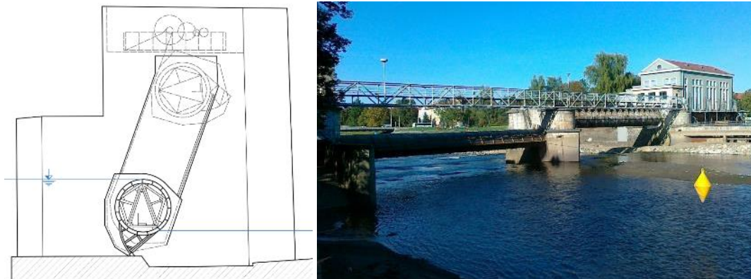
Obr. 4.110: Válcový jez. Schéma Radka Račoch a Michaela Mrvová, 2021 (upraveno dle: Průcha, 1980). Vpravo Jiráskův jez v Českých Budějovicích. Foto Archiv VUT, 2017.
