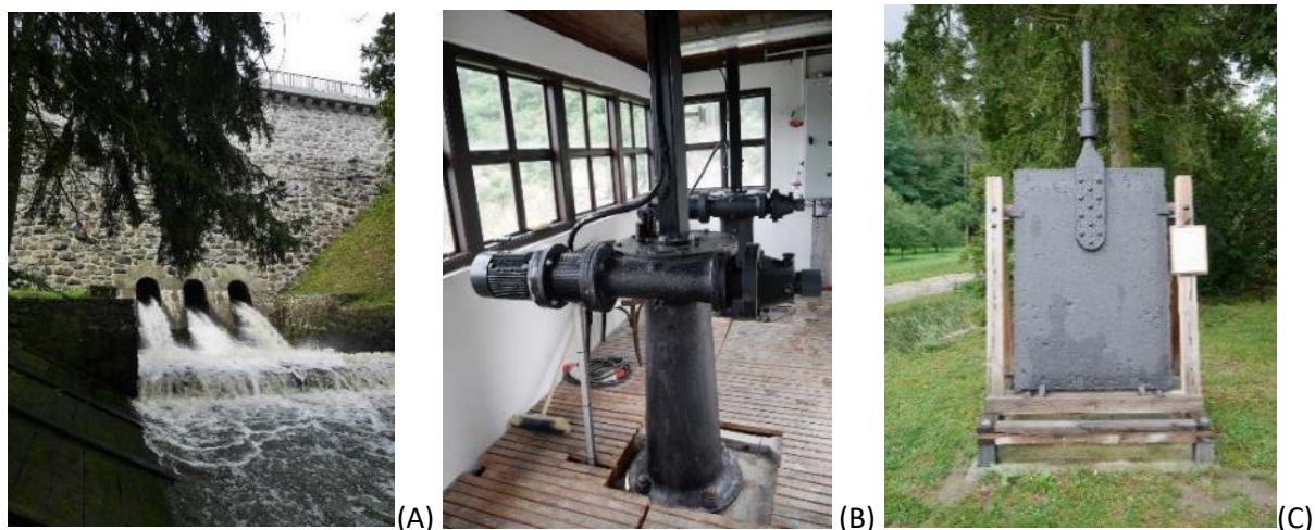
Obr. 4.25: Přehrada Jevišovice (1884–1896) – zděná tížná přehrada. (A) spodní výpusti přehrady, které představují tři štoly; (B) ovládání provozních uzávěrů spodních výpustí umístěné na koruně hráze, původně nekryté, teprve dodatečně byl nad ním vybudován objekt; (C) jeden z původních uzávěrů výpusti, umístěný dnes pod přehradou. Foto Michaela Ryšková, 2020.
