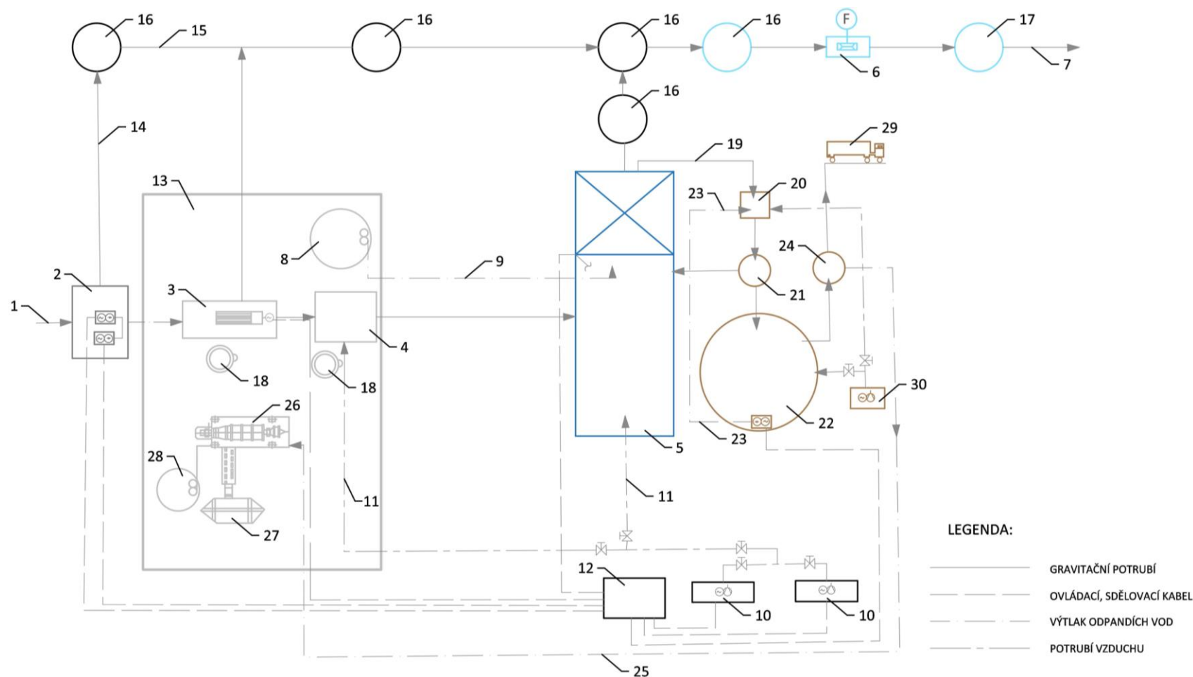
Obr. 4.265: Technologické schéma (linka) ČOV pro obec do 2000 obyvatel (Starovice, okres Břeclav): 1 – nátok, 2 – čerpací stanice, 3 – česle, 4 – lapák písku a tuku, 5 – aktivace, 6 – měřící objekt na odtoku + Parshallův žlab, 7 – odtok do vodního toku (recipientu), 8 – zásobník na srážedlo fosforu, 9 – potrubí pro dopravu srážedla, 10 – dmýchárna, 11 – přívod vzduchu do aktivace, nebo k lapáku, 12 – řídicí jednotka aktivace, 13 – provozní objekt, 14 – havarijný přepad surové vody, 15 – havarijný gravitační obtok ČOV, 16 – provozní a kontrolní šachtice, 17 – kontrolní šachtice na odtoku, 18 – popelnice na shrabky, 19 – vratný kal, 20 – čerpací stanice kalu, 21 – šachtice, 22 – kalojem, 23 – kalová voda, 24 – šachtice, 26 – dehydrátor kalu, 27 – kontejner na odvoz kalu, 28 – zásobník flokulantu na kal, 29 – odtah přebytečného kalu a možnost odvozu, 30 – dmychadlo. Schéma Radka Račoch a Michaela Mrvová, 2021 (upraveno dle: poskytnuté projektové dokumentace).
