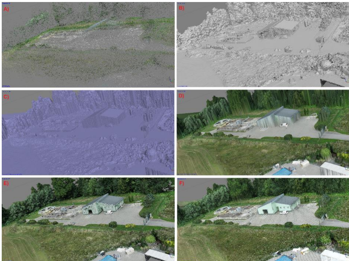
Obr. 4.270: Geneze 3D modelu malé ČOV v jednotlivých krocích: (A) identifikace společných bodů na jednotlivých fotografiích; (B) vytvoření mračka bodů; (C) vytvoření drátového modelu; (D) přiřazení barevné
