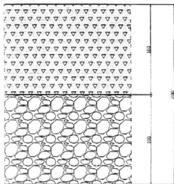
podkladní vrstva vozovky
