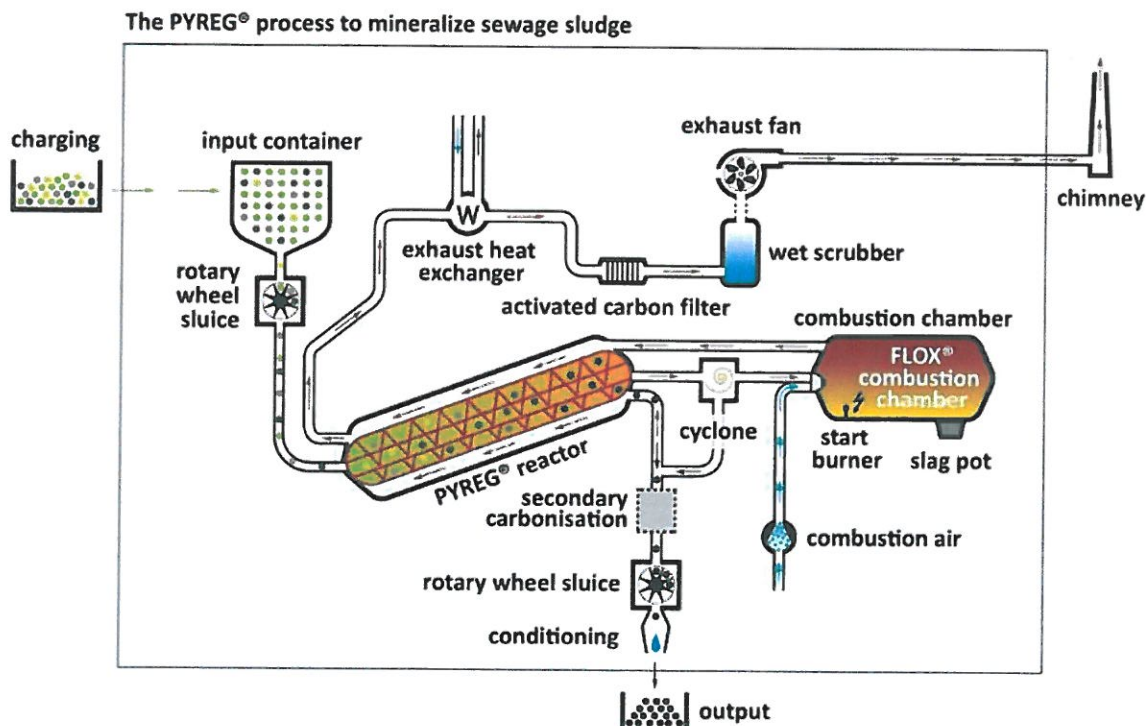
Obr. 1 Schéma technologické linky na výrobu biocharu [1]
