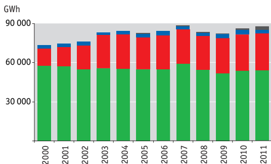
Graf 1 → Výroba elektřiny podle druhu elektráren v ČR [GWh], 2000–2011
