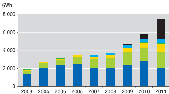
Graf 1 → Výroba elektřiny z OZE v ČR [GWh], 2003–2011
