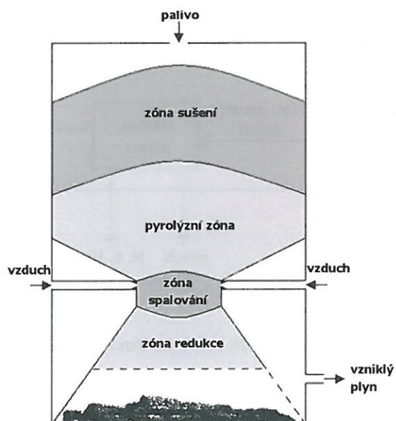
Obr. 4: Schematické znázornění souproutého generátoru Imbert
