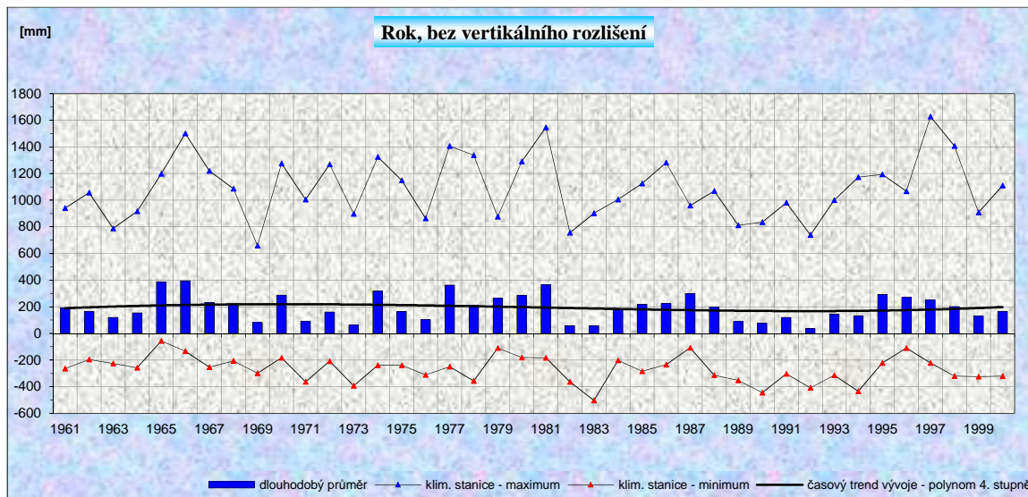
Obr. 3: Vláhová bilance travního porostu, území ČR bez rozlišení výškových pásem, průměrné, maximální a minimální úhrny za rok a vegetační období (1961–2000)
