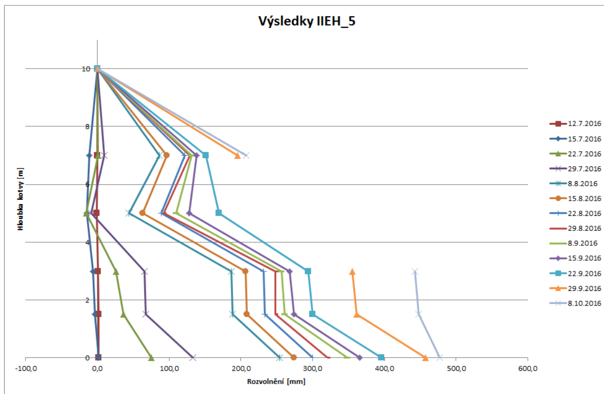
Obr. 5.29 Graf rozvolnění uhlého pilíře x hloubka kotvy – extenzometr IIEh5.
