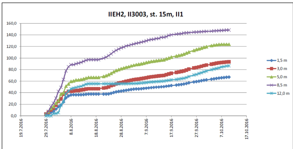
Obr. 5.14 Graf rozvoľnění uhelného pilíře – extenzometr IIEh2.
