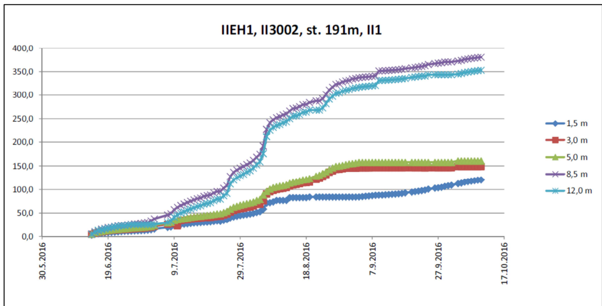
Obr. 5.13 Graf rozvoľnění uhelného pilíře – extenzometr IIEh1
