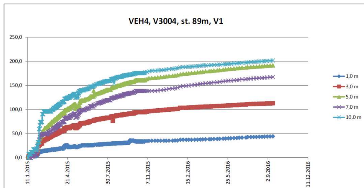
Obr. 4.27 Graf rozvolnění uhlého pilíře – extenzometr VEh4.
