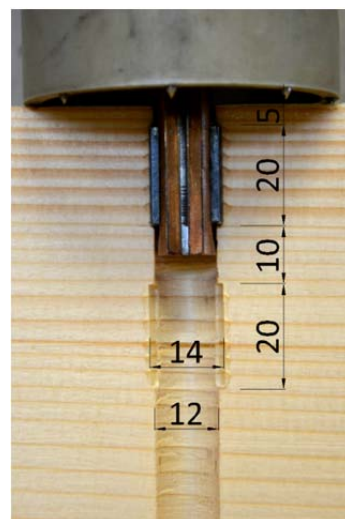
Obr. 5 Detail táhla s rozevíracím klínem a zakulacenými čelistmi (Kloiber a Drdácěk, 2015)
