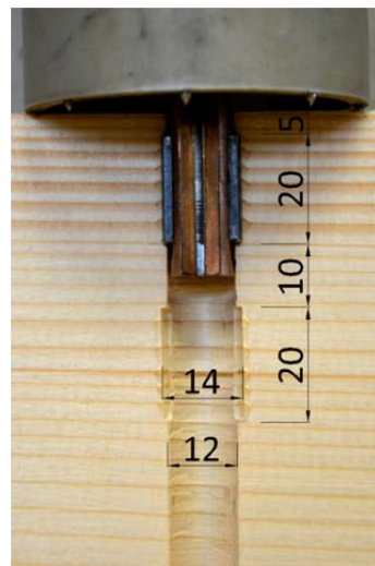
Obr. 5 Detail táhla s rozevíracím klínem a zakulacenými čelistmi (Kloiber a Drdácák, 2015)
