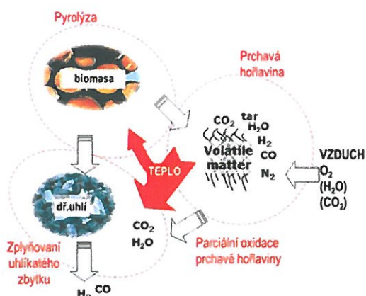
Obr. 1: Zjednodušené schéma procesu zplyňování biomasy [1]
