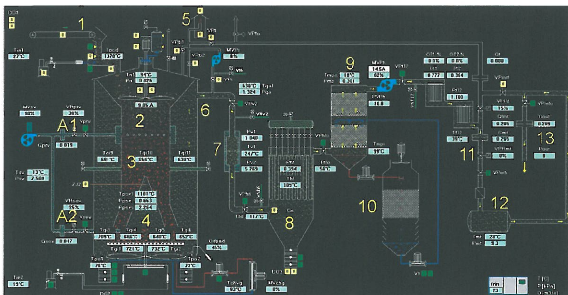
1- vstup paliva do GP750, 2-dosušovací část, 3- pyrolýzní část, 4- parciálně-oxidační část, 5-spalovací fléra, 6-odvod plynu z generátoru 7- vodní chladič plynu, 8- rukávové látkové filtry, 9- kontaktní chlazení plynu, 10- kontaktní chlazení plynu v chladiči věže, 11-měřicí clona,
