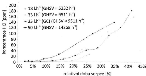
Obr. 1 – Závislost výstupní koncentrace HCl na stupni využití sorbentu pro různé prostorové rychlosti. (Pro měření byl použit sorbent skládající se z Na a nosiče. Nosičem byla \gamma -alumina s obchodním názvem Condea. Pracovalo se při konstantním složení plynu 240 ppm v HCl, 38 obj. % H 2 O a 62 obj. % N 2 . Objem sorbentu byl 10 ml a výška vrstvy sorbentu byla 6,5 cm. t_{sorpce} = 500 °C, p = cca 1 bar). [23]
