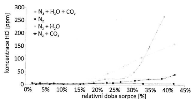
Obr. 2 – Závislost výstupní koncentrace HCl na stupni využití sorbentu pro různé plyny. (Pro měření byl použit sorbent skládající se z Na a nosiče. Nosičem byla \gamma -alumina s obchodním názvem Condea. Pracovalo se při konstantním složení plynu 240 ppm v HCl, 38 obj. % H 2 O + CO 2 a 62 obj. % N 2 . Prostorová rychlost byla 9 000 h -1 (500 °C). Objem sorbentu byl 10 ml a výška vrstvy sorbentu byla 6,5 cm. t_{sorpce} = 500 °C, p = cca 1 bar). [23]
