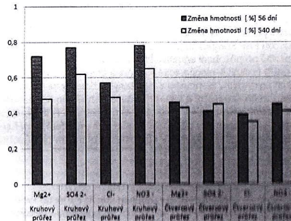
Obr. 2 Změna hmotnosti FRP vzorků po 56 a 540 dnech v agresivním prostředí
