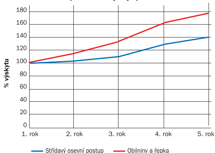
Vliv střídání plodin na výskyt pcháče rolního
