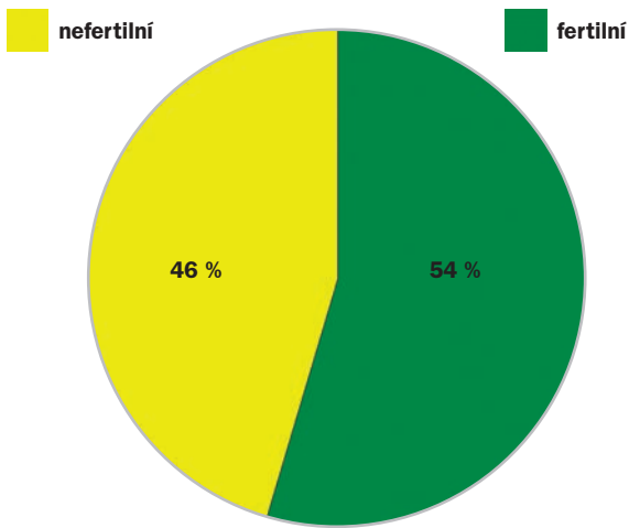
Podíl fertálních a nefertálních nažek v úbořech pcháče rolního
