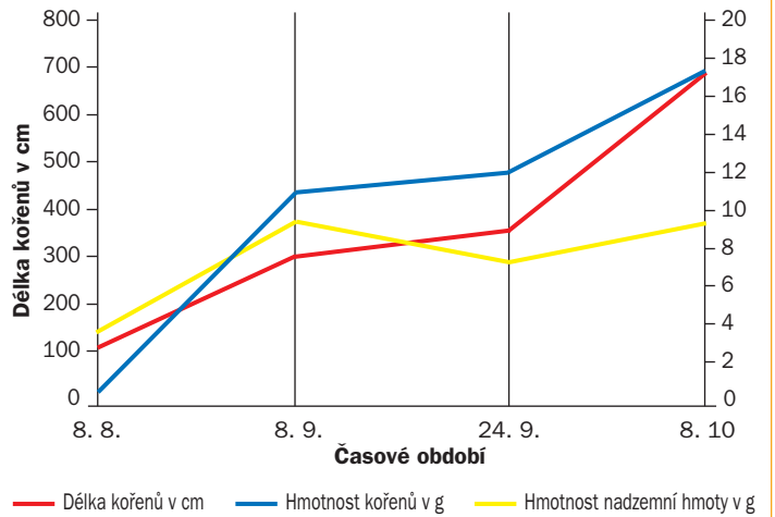
Přírůstky nadzemní a podzemní hmoty Cirsium arvense (L.) Scop. – nádobový pokus
