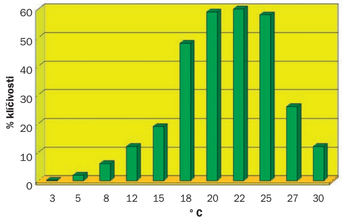
Klíčivost nažek pcháče rolního v závislosti na teplotě
