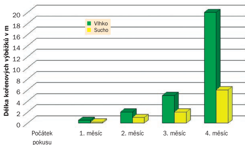
Vliv vláhy na tvorbu kořenových výběžků pcháče rolního
