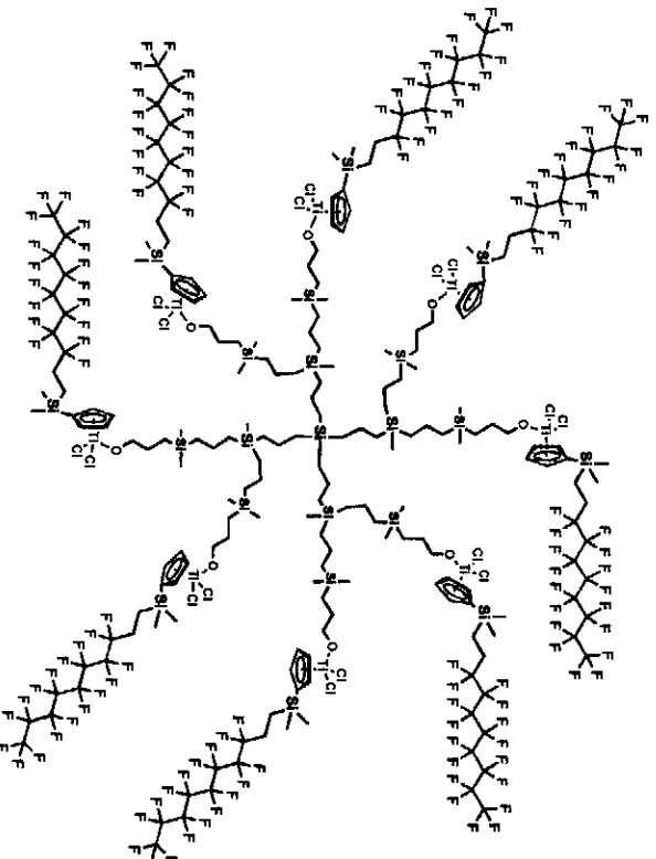
Periferně fluorovaný metalodendrimer s osmi perfluoroketonylovými skupinami
