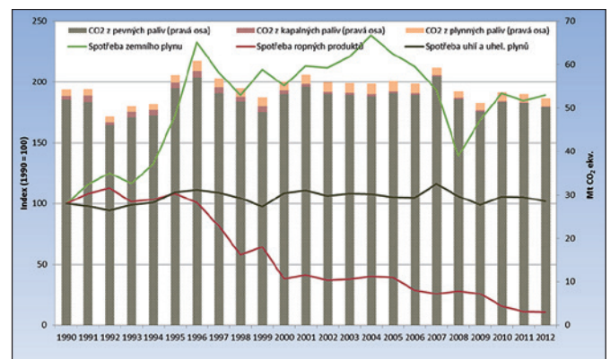
Obr. 5. Emise skleníkových plynů ze spalování pevných, kapalných a plyných paliv a spotřeba pevných, kapalných a plyných paliv ve veřejné energetice a výrobě tepla v ČR [index: 1990 = 100, Mt CO 2 ekv.] 1990–2012
