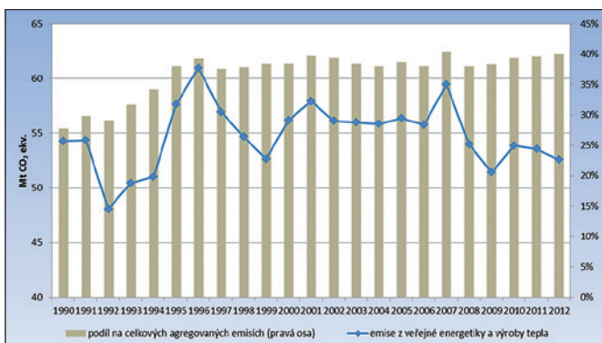
Obr. 3. Emise skleníkových plynů z veřejné energetiky a výroby tepla v ČR a podíl veřejné energetiky na celkových agregovaných emisích [Mt CO 2 ekv., %] 2000–2012
