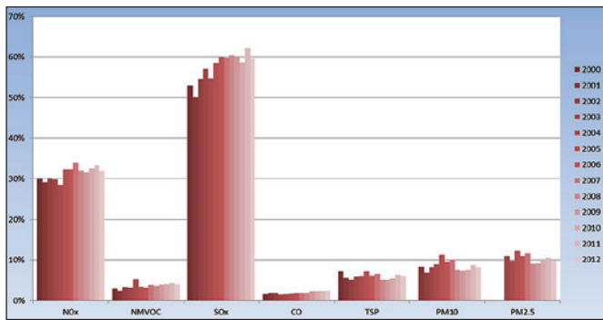
Obr. 10. Vývoj podílu veřejné energetiky a výroby tepla na celkových emisích znečišťujících látek v ČR [%] 2000–2012
